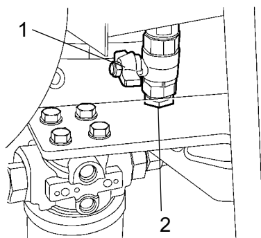
Fig. Lato sottostante del serbatoio idraulico 1. Rubinetto di drenaggio 3. Tappo
