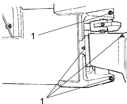
Fig. Snodo, lato destro 1. Ingrassatori, snodo (4)
