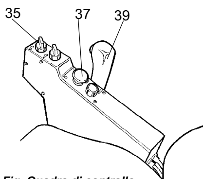
Fig. Quadro di controllo 35. Selettore di velocità 37. Pulsante del freno di riserva/parcheggio 39. Leva di marcia avanti/indietro
