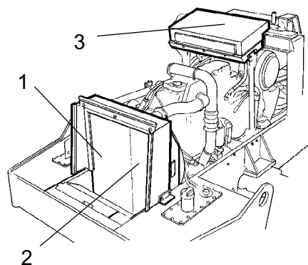
Rys. Komora silnika 1. Chłodnica wody 2. Chłodnica świeżego powietrza 3. Chłodnica płynu hydraulicznego
