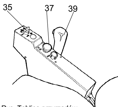
Rys. Tablica przyrządów 35. Przełącznik prędkości 37. Pokrętło hamulca rezerwowego/postojowego 39. Dźwignia jazdy do przodu/do tyłu
