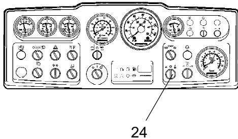
Rys. Tablica przyrządów 24. Przełącznik amplitudy niska/0/wysoka
