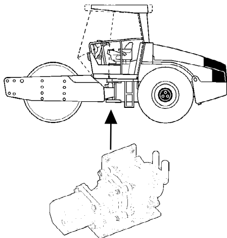
Rys. Sprężarka
