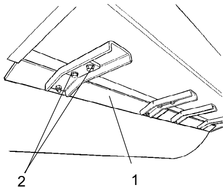
Rys. Skrobaki 1. Łopatką skrobaka (x4) 2. Śruby
