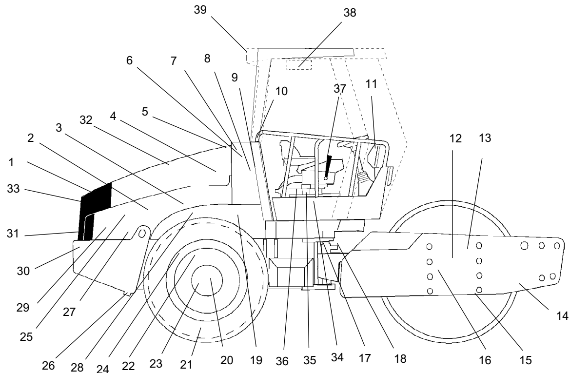
Rys. Punkty serwisowania i konserwacji
