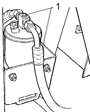
Rys. Filtr osuszający 1. Wziernik
