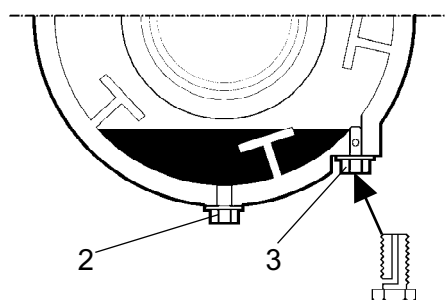
Rys. Kasetę bębna 2. Kurek spustowy 3. Kurek poziomy
