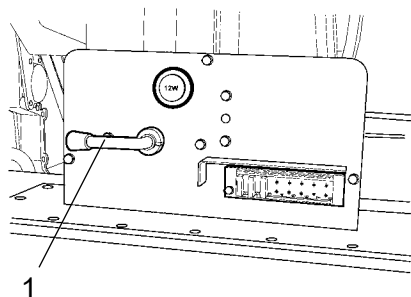
Εικ. Πλαίσιο ελκυστήρα, πίσω αριστερά 1. Γενικός διακόπτης
