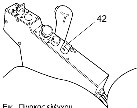
Εικ. Πίνακας ελέγχου 42. Φρένο στάθμευσης
