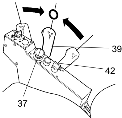
Εικ. Πίνακας ελέγχου 37. Διακοπή λειτουργίας έκτακτης ανάγκης 39. Μοχλός κίνησης προς τα εμπρός/όπισθεν 42. Κουμπί φρένου στάθμευσης
