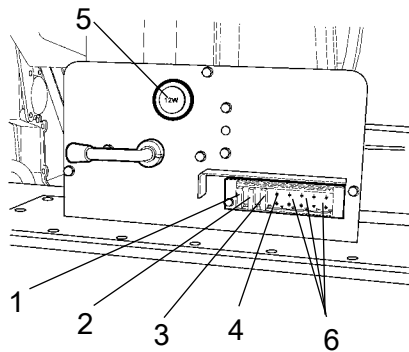
Εικ. Διαμέρισμα κινητήρα 1. Κινητήρας QSB (ανάφλεξη) 2. Λυχνίες συστήματος διάγνωσης κινητήρα 3. Ηλεκτρονικά εξαρτήματα ECM 4. Ασφάλεια, Πρίζα 12V 5. Πρίζα 12V 6. Εφεδρικό
