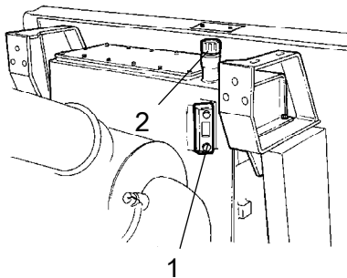
Εικ. Ρεζερβουάρ υδραυλικού συστήματος 1. Γυάλινη θυρίδα ελέγχου 2. Σωληνάκι πλήρωσης
