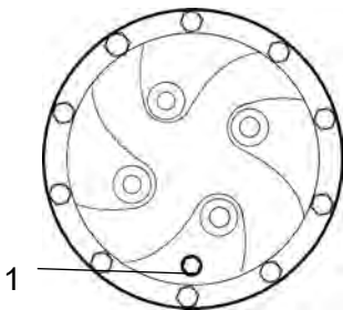
Εικ. Πλανητικό σύστημα γραναζιών/θέση αποστράγγισης
