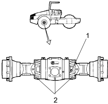
Εικ. Οπίσθιος άξονας
