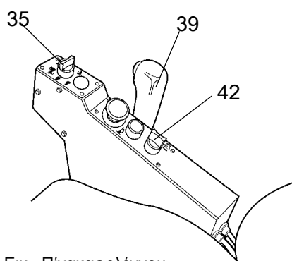
Εικ. Πίνακας ελέγχου 35. Επιλογέας ταχύτητας 39. Μοχλός κίνησης προς τα εμπρός/όπισθεν 42. Κουμπί φρένου στάθμευσης
