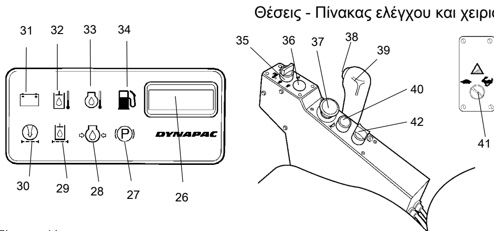
Εικ. Πίνακας ελέγχου
