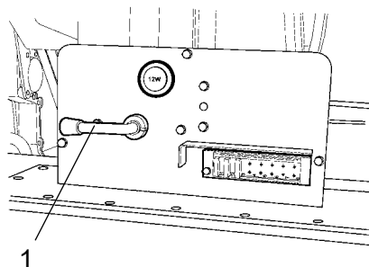
Fig. Telaio della macchina: lato posteriore sinistro 1. Interruttore principale
