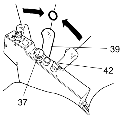
Fig. Quadro di comando 37. Arresto di emergenza 39. Leva di marcia avanti/indietro 42. Pulsante del freno di parcheggio
