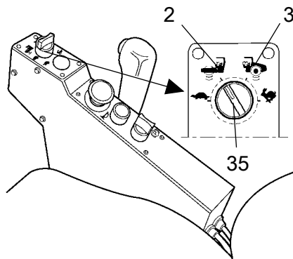
Fig. Quadro di controllo 35. Selettore di velocità 2. Posizione 2 3. Posizione 3
