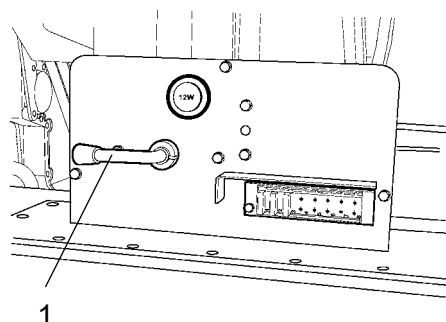
Fig. Vano motore 1. Interruttore principale
