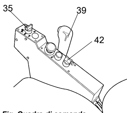
Fig. Quadro di comando 35. Selettore di velocità 39. Leva di marcia avanti/indietro 42. Pulsante del freno di parcheggio
