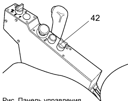
Рис. Панель управления 42. Рукоятка стояночного тормоза
