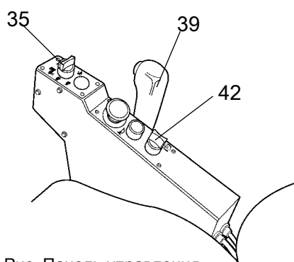
Рис. Панель управления 35. Переключатель скоростей 39. Рычаг прямого/обратного хода 42. Рукоятка стояночного тормоза
