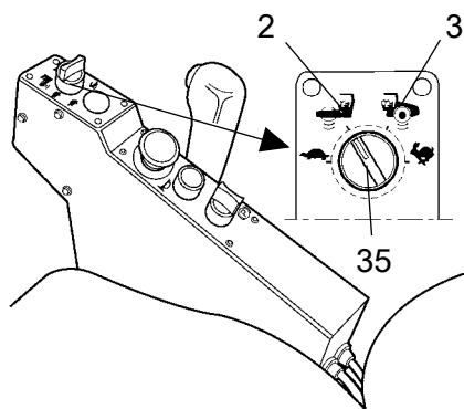
Рис. Панель управления 35. Переключатель скоростей 2. Положение 2 3. Положение 3
