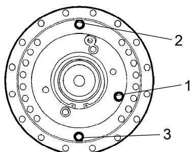
Рис. Проверка уровня масла - валец
