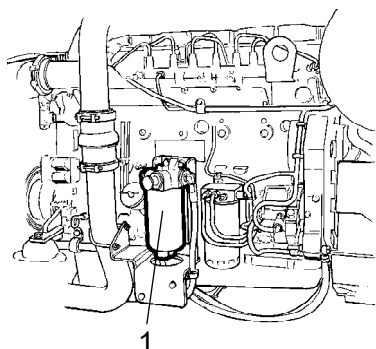
Рис. Отделение двигателя 1. Предварительный фильтр топлива
