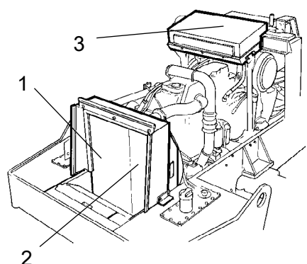
Рис. Отделение двигателя 1. Водяной радиатор 2. Охладитель наддувочного воздуха 3. Радиатор гидравлической жидкости
