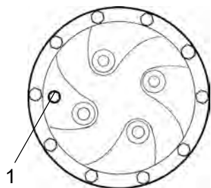
Рис. Планетарная передача/положение наполнения 1. Пробка
