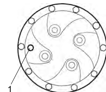
Рис. Проверка уровня - Планетарная передача 1. Уровень/пробка заливного отверстия
