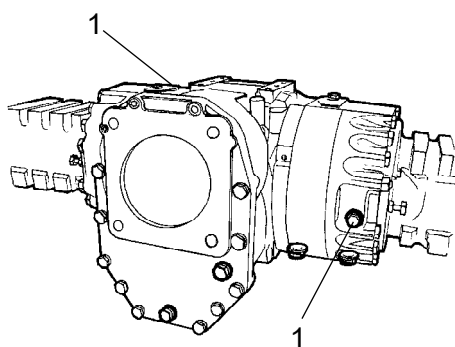
Рис. Проверка уровня - корпус дифференциала
