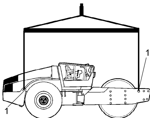
Рис. Подготовленный к подъему каток 1. Табличка подъема
