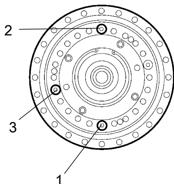
Рис. Коробка передач вальца 1. Пробка сливного отверстия 2. Пробка заливного отверстия 3. Пробка уровня
