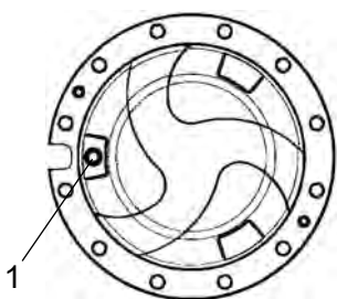
Рис. Планетарная передача/положение заполнения 1. Пробка
