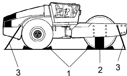
Рис. Транспортировка 1. Колодка 2. Блок 3. Вязочная проволока
