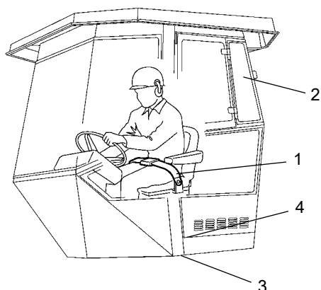
Рис. Рабочее место оператора
