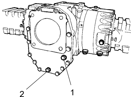
Рис. Коробка отбора мощности 1. Пробка заливного отверстия / отверстия для определения уровня 2. Пробка сливного отверстия
