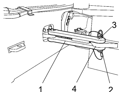
Рис. Шарнирное сочленение в заблокированном положении 1. Фиксатор 2. Стопорный штифт 3. Запорный рычаг 4. Стопорный выступ
