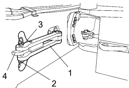
Рис. Шарнирное сочленение в открытом положении 1. Фиксатор 2. Стопорный штифт 3. Запорный рычаг 4. Стопорный выступ
