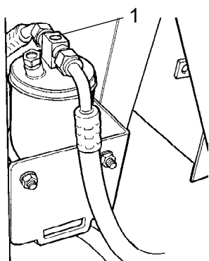
Рис. Осушивающий фильтр 1. Смотровое окно
