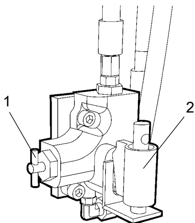
Рис. Насос для освобождения тормоза 1. Ручка для приведения тормоза в действие 2. Рычаг насоса
