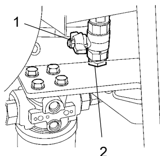
Рис. Нижняя сторона бака гидравлической системы 1. Кран сливного отверстия 2. Заглушка
