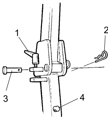
Fig. Meccanismo di bloccaggio ROPS 1. Vite di tensionamento 2. Spina 3. Dente 4. Respingente in gomma
