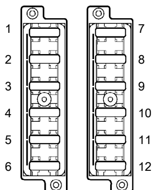
Rys. Skrzynki bezpieczników, lewa i prawa strona
