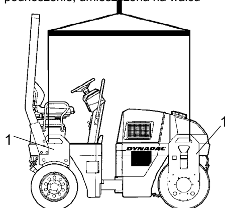
Rys. Podnoszenie walca
