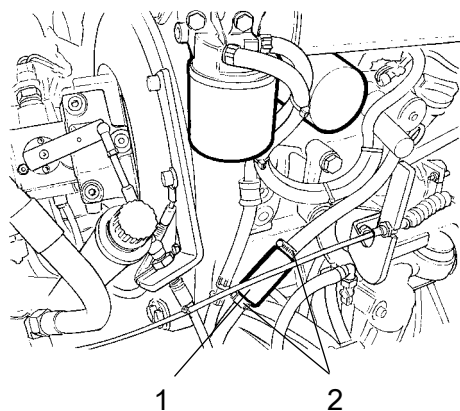
Fig. Compartimento do motor 1. Pré-filtro 2. Braçadeiras de mangueira
