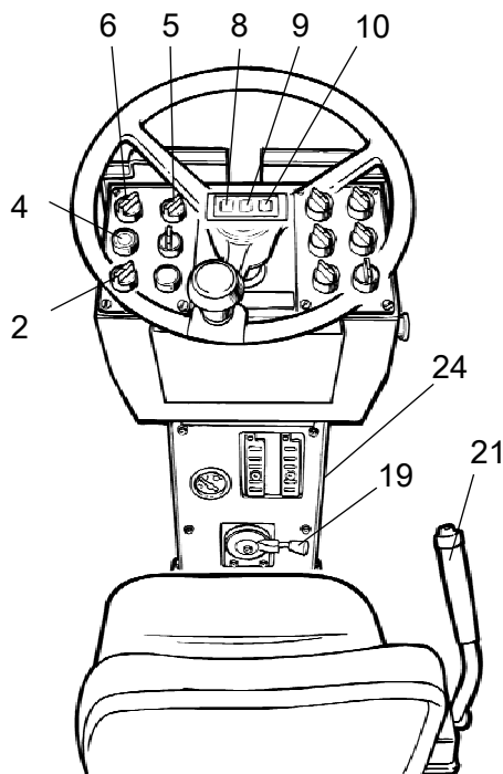
Fig. Coluna de instrumentos 2. Interruptor de arranque 4. Interruptor de arranque 5. Interruptor de vibração 6. Botão do travão de estacionamento 8. Lâmpada de carga 9. Lâmpada de aviso dos travões 10. Lâmpada da pressão do óleo/Temperatura do motor 19. Comando da rotação do motor 21. Comando de Avanço/Recuo 24. Paragem de emergência
