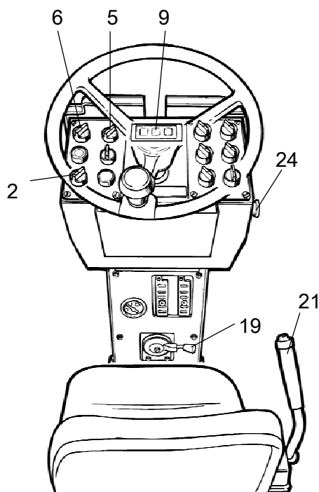
Fig. Painel de comando 2. Interruptor de arranque 5. Interruptor de vibração 6. Botão do travão de estacionamento 9. Lâmpada de aviso dos travões 19. Comando da rotação do motor 21. Comando de avanço/recuo 24. Paragem de emergência
