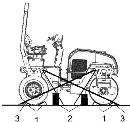
Rys. Ustawienie 1. Kliny 2. Kliny drewniane 3. Pasy
