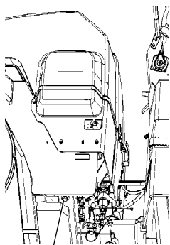
Rys. Lewa strona ramy 1. Korek spustowy
