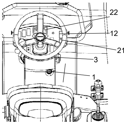
Rysunek. Tablica przyrządów 1. Przełącznik rozrusznika 3. Hamulec awaryjny 12. Przełącznik, zraszanie 21. Przełącznik, zraszanie kół 22. Panel ostrzegawczy
