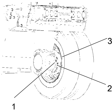
Rys. Lewa strona bębna 1. Okładzina hamulca 2. Wkręt mocujący 3. Nakrętka odłączania
