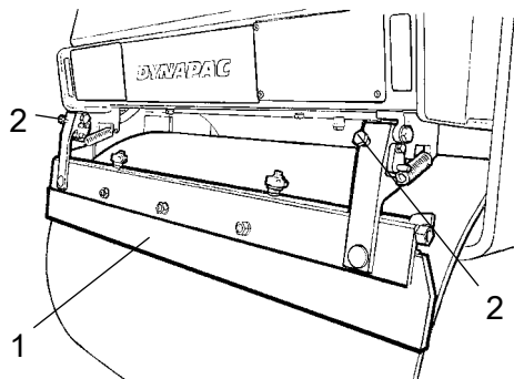
Rys. Skrobaki sprężynowe 1. Ostrze skrobaka 2. Śruby regulacyjne
