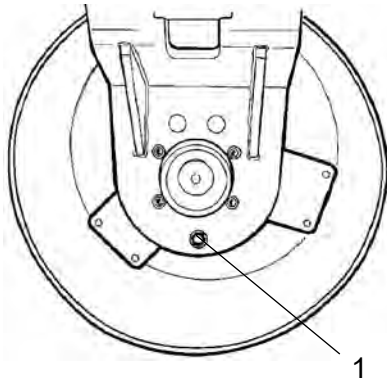
Fig. Cilindro, lado da vibração 1. Bujão de drenagem
