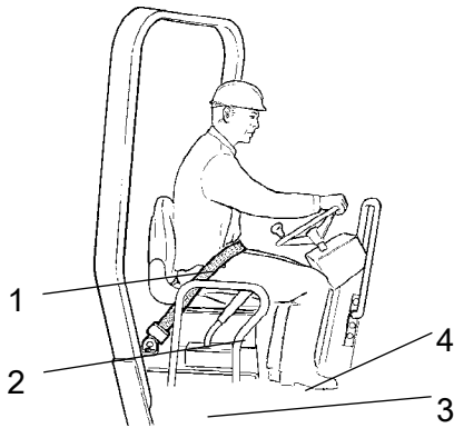
Fig. Assento do condutor 1. Cinto de segurança 2. Corrimões de segurança 3. Elemento de borracha 4. Protecção contra escorregamento
