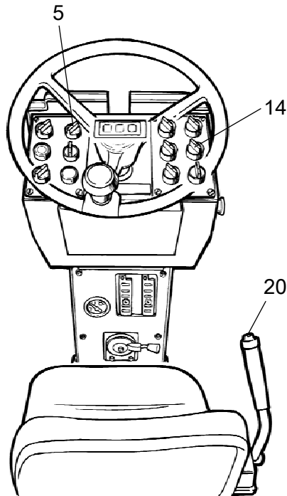
Fig. Coluna de instrumentos 5. Chave da vibração 14. Vibração cilindro dianteiro/traseiro (Opcional) 20. Comutador da vibração
