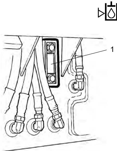
Fig. Reservatório de óleo hidráulico 1. Visor de nível
