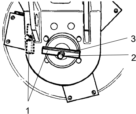
Fig. Lado esquerdo do cilindro
