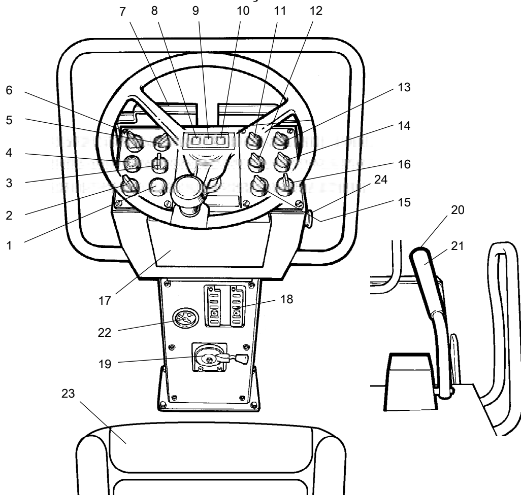
Fig. Instrumentos e painel de controle
