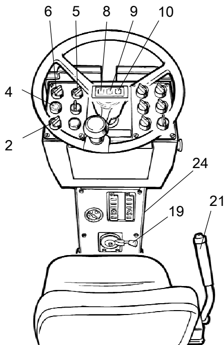
Fig. Coluna de instrumentos
