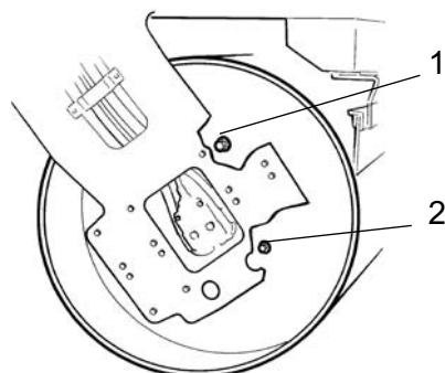
Фиг. Вибрираща страна на барабана 1. Пробка за пълнене 2. Контролна пробка за нивото
