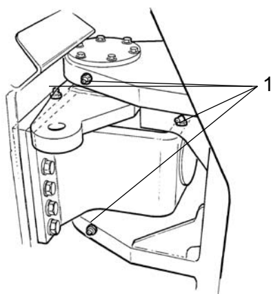
Фиг. Дясна страна на шарнира 1. Гресьорки
