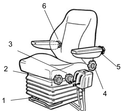
Фигура. Седалка на оператора 1. Лостче - регулировка по дължина 2. Колелце - регулировка по височина 3. Колелце - наклон на възглавницата на седалката 4. Колелце - регулировка на наклона на облегалката 5. Колелце - регулировка на наклона на подлакътника 6. Колелце - регулировка на опората за кръста
