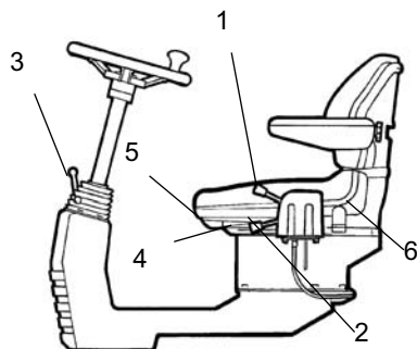
Фигура. Позиция на оператора 1. Блокиращ лост - напречен ход 2. Блокиращ лост - завъртане 3. Блокиращ лост - ъгъл на кормилната колона 4. Блокиращ лост - настройка на дължина 5. Лостче - наклон на облегалката 6. Лостче - настройка на теглото
