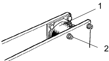
Фиг. Барабан, страна на вибрацията 1. Гумен елемент 2. Затягащи винтове
