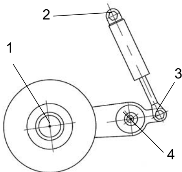
Фиг. Четири точки за гресиране на ръбовите фрези
