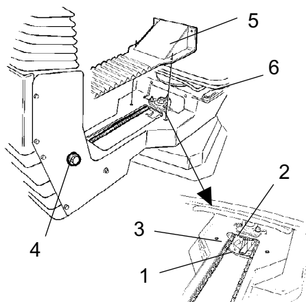
Фиг. Лагер на седалка 1. Гресьорка 2. Зъбно колело 3. Водеща верига 4. Регулиращ винт 5. Капак 6. Релси за плъзгане на седалката
