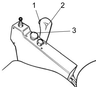
Фиг. Контролно табло 1. Превключвател Вкл/Изкл вибрация 2. Лост преден/заднен ход 3. Бутон за аварийна/ръчна спирачка
