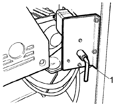
Фигура. Място за акумулатора (врата отляво на двигателя) 1. Главен прекъсвач
