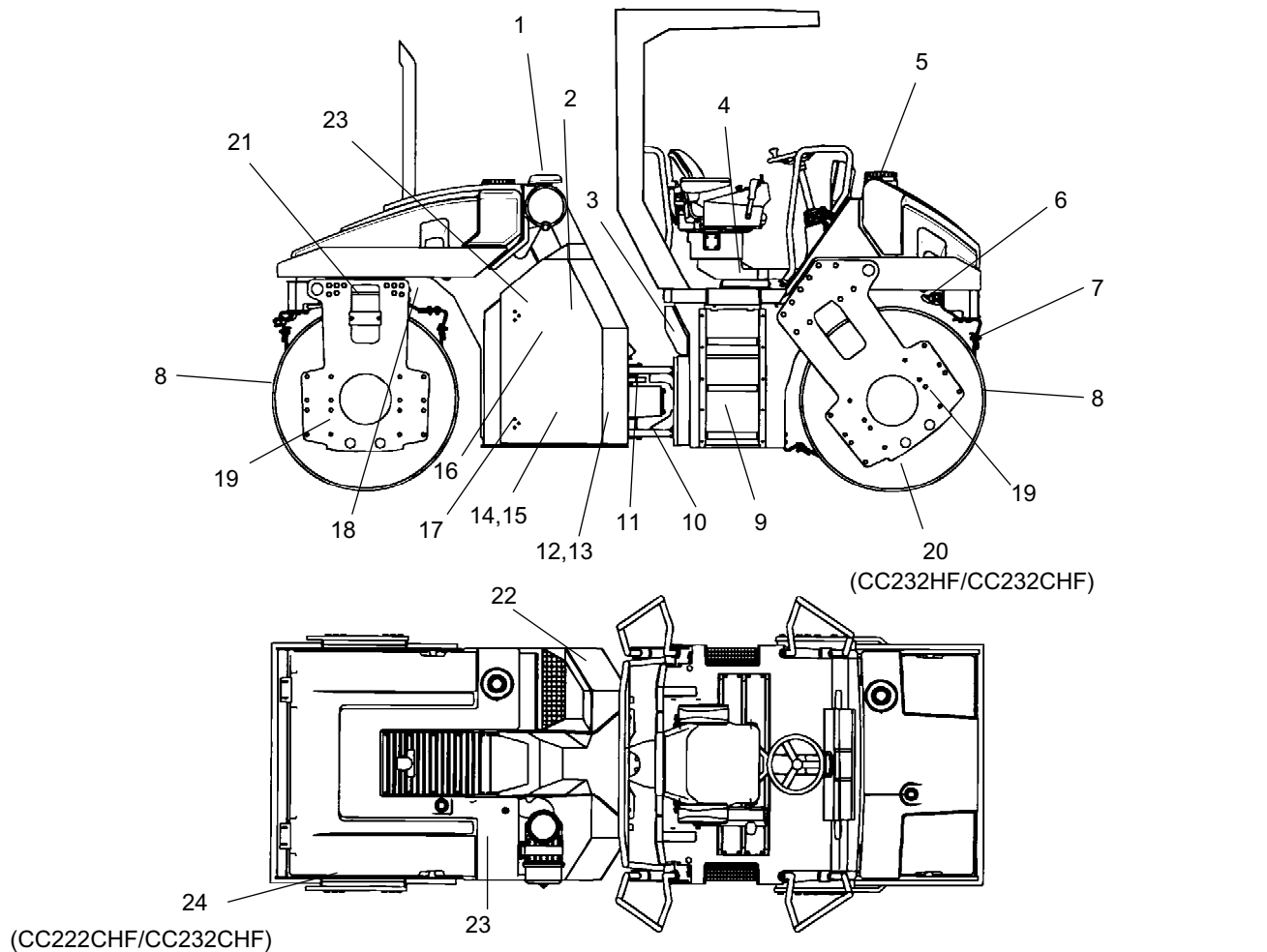
Фигура. Точки на обслужване и поддръжка
