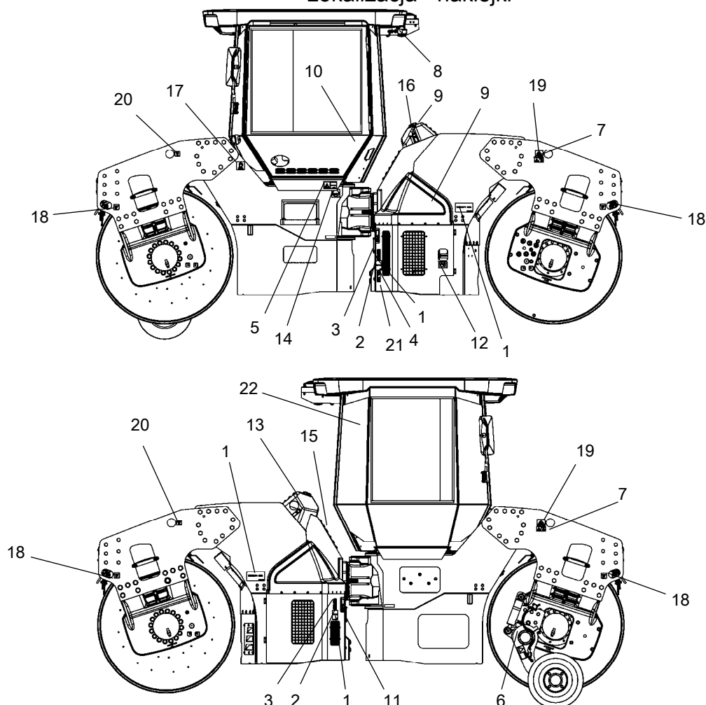
Rys. Lokalizacja, naklejki i znaki
