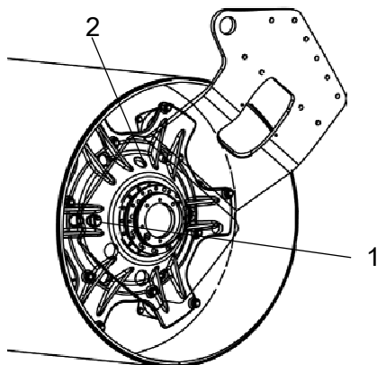
Rys. Sprawdzenie poziomu oleju - przekładnia bębna 1. Korek poziomu 2. Korek napełniania
