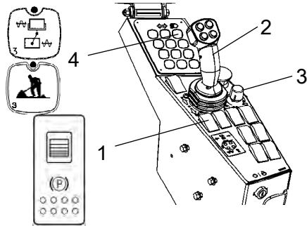
Rys. Panel sterowania
