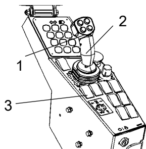
Rys. Panel sterowania 1. Przełącznik włączania/wyłączania wibracji 2. Dźwignia jazdy do przodu / do tyłu 3. Przycisk hamulca postojowego
