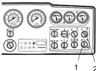
Kuva: Vaihtokytkin
