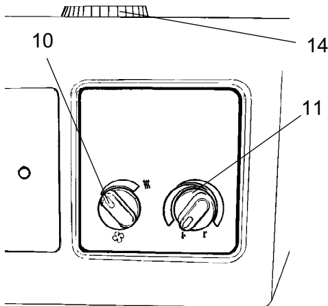
Kuva: Ohjaamo takaa, varustettu lämmittimellä
