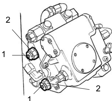
Kuva: Vetopumppu
