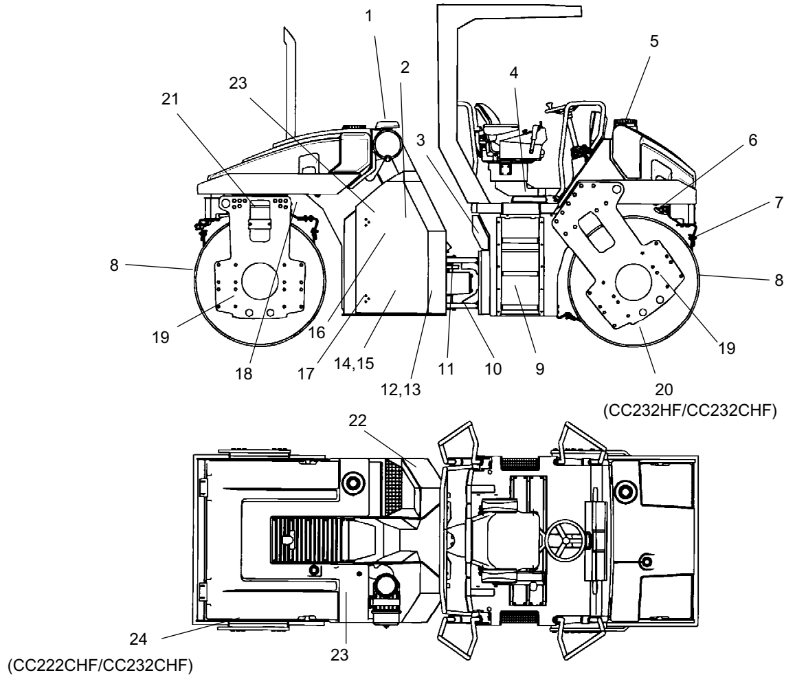
Kuva: Huolto- ja tarkastuskohteet
