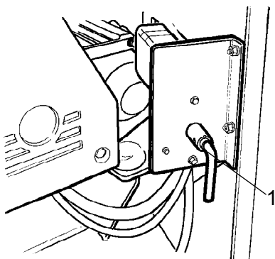
Kuva: Akkukotelo (moottoritilan vasen luukku) 1. Päävirtakytkin
