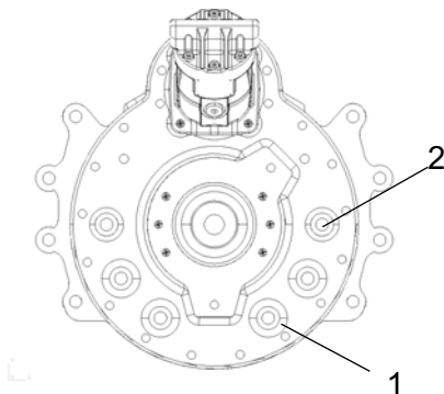
Kuva: Valssin vaihteisto 1. Tyhjennystulppa 2. Täyttötulppa/tasotulppa
