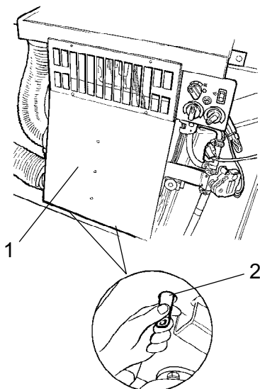
Kuva: Ilmastointi 1. Jäähdytyselementti 2. Tyhjennysventtiili
