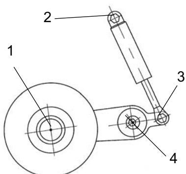
Kuva: Reunaleikkurin neljä voitelukohdetta
