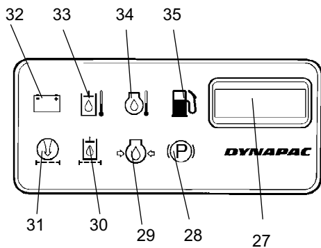
Kuva: Kojetaulu
