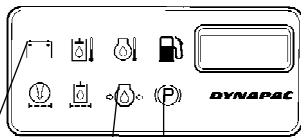
Kuva: Kojetaulu 2. Latausmerkkivalo 3. Öljynpaineen merkkivalo 4. Jarrumerkkivalo
