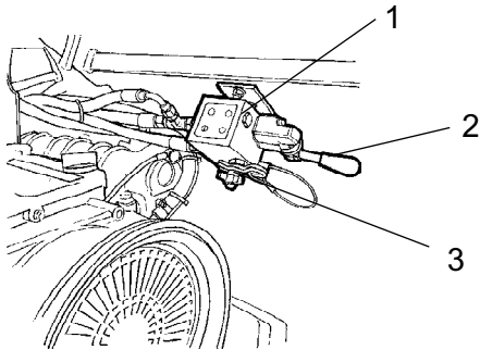
Kuva: Jarrujen vapauttamisventtiili
