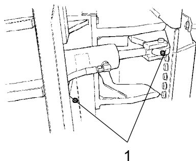
Kuva: Ohjausnivelen vasen puoli 1. Voitelunipat
