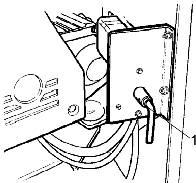
Kuva: Akkukotelo (moottoritilan vasen luukku) 1. Akun eristyskytkin
