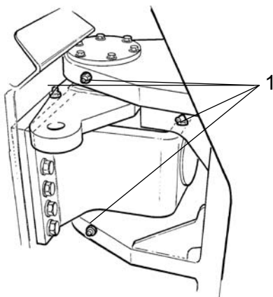
Kuva: Ohjausnivelen oikea puoli 1. Voitelunipat
