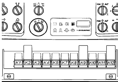
Kuva: Mittaritaulu
