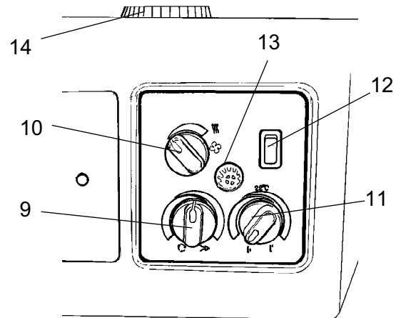
Kuva: Ohjaamo takaa, ilmastointilaitte (lisävaruste)
