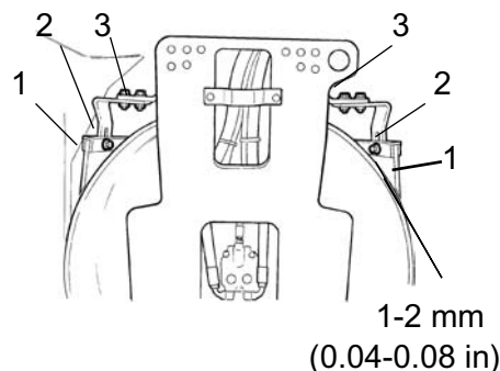
Fig. Bakre valsskrapor 1. Skrapblad 2. Justerskruvar 3. Justerskruvar
