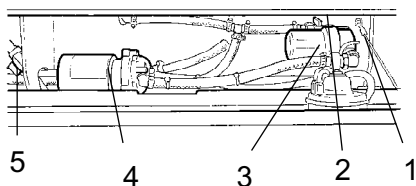
Fig. Pumpsystem 1. Grovfilter 2. Avstängningskran 3. Filterhus 4. Vattenpump 5. Dräneringskran
