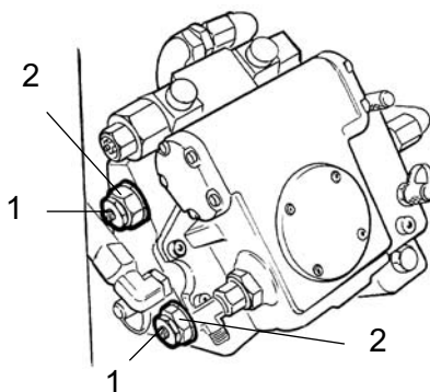
Fig. Framdrivningspump
