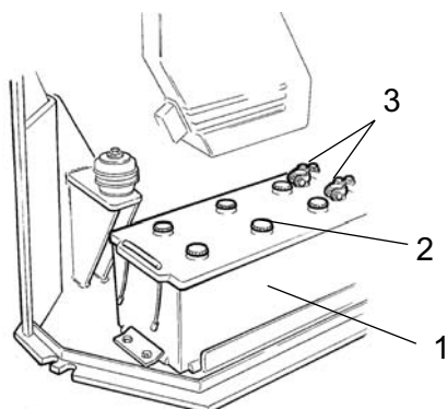
Fig. Batteriutrymme
