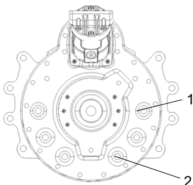
Fig. Nivåkontroll - valsväxellåda 1. Nivåplugg 2. Avtappningsplugg
