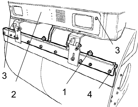
Fig. Främre vals 1. Munstycke 2. Pumpsystem/lucka 3. Snabbskruvar 4. Dräneringsplug
