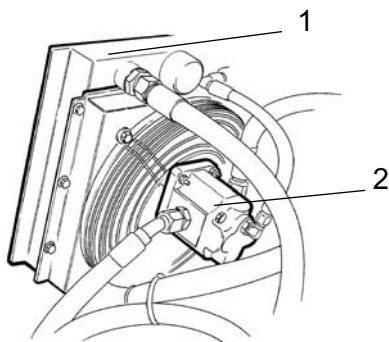
Fig. Hydrauloljekylare
