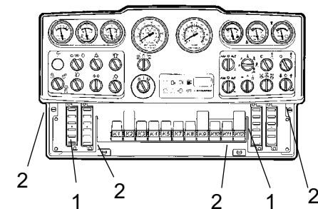
Fig. Instrumentpanel 1. Säkringsdosor 2. Snabbskruvar
