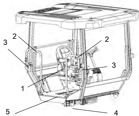
Fig. Position du conducteur
