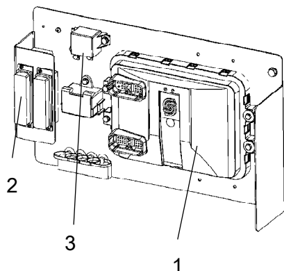
Fig. Central électrique principal
