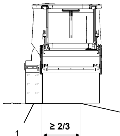
Fig. Position des rouleaux pour la conduite le long des bords 1. Pivot d'articulation centrale
