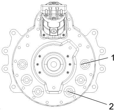
Fig. Contrôle de niveau d'huile - réducteur de cylindre 1. Bouchon de niveau 2. Bouchon de vidange
