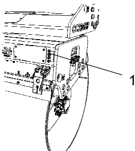
Rys. Bęben tylny 1. Cztery smarowniczk
