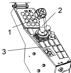
Rys. Panel sterowania 1. Przełącznik włączania/wyłączania wibracji 2. Dźwignia jazdy do przodu / do tyłu 3. Przycisk hamulca postojowego
