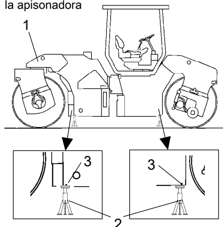
Figura. Apisonadora elevada con un gato
