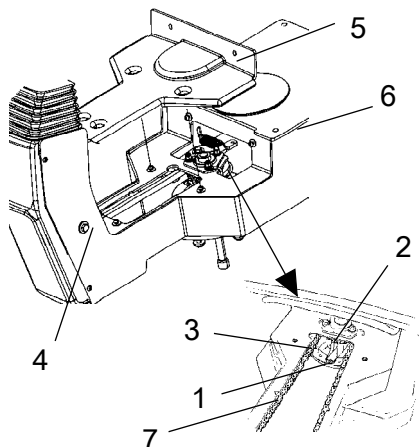
Figura. Cojinete del asiento 1. Engrasador 2. Rueda del engranaje 3. Cadena de dirección 4. Tornillo de ajuste 5. Cubierta 6. Raíles deslizantes 7. Marcas
