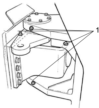
Rys. Prawa strona połączenia przegubowego 1. Smarowniczki
