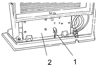
Rys. Przedział akumulatora 1. Przełącznik odcinający akumulatora 2. Tablica bezpieczników głównych
