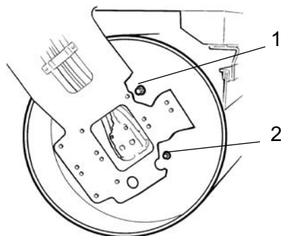
Rys. Bęben, strona wibracji 1. Korek wlewu 2. Korek poziomu
