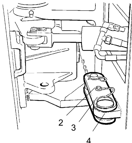
Rys. Połączenie przegubowe w położeniu odblokowanym
