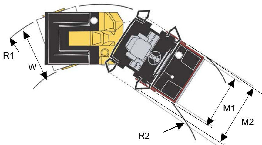
Wymiary, widok od góry
