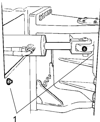
Rys. Lewa strona połączenia przegubowego 1. Smarowniczki
