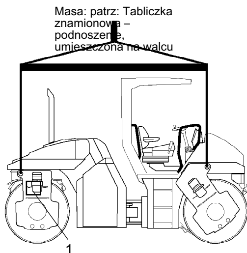
Rys. Walec przygotowany do podnoszenia 1. Tabliczka znamionowa - podnoszenie
