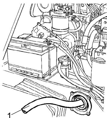
Fig. Bränsletank
