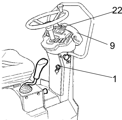
Fig. Instrumentpanel 1. Startströmbrytare 9. Instrumentskydd 22. Panel för varningslampor
