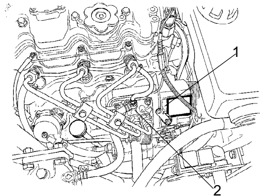
Fig. Motor 1. EPA-skylt (USA) 2. Typskytt
