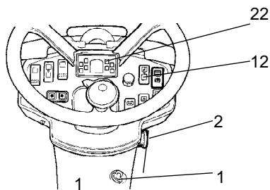
Fig. Instrumentpanel 1. Startströmställare 2. Nödbroms 12. Strömställare bevvatning 22. Varningspanel
