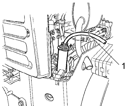
Fig. Hydrotank 1. Avtappning
