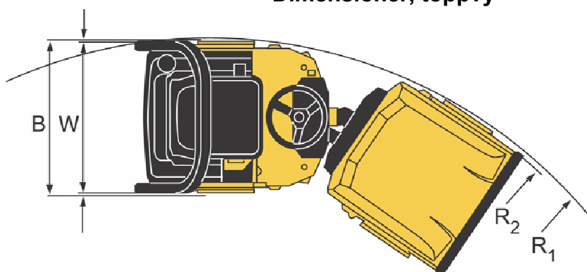
Dimensioner, toppvy
