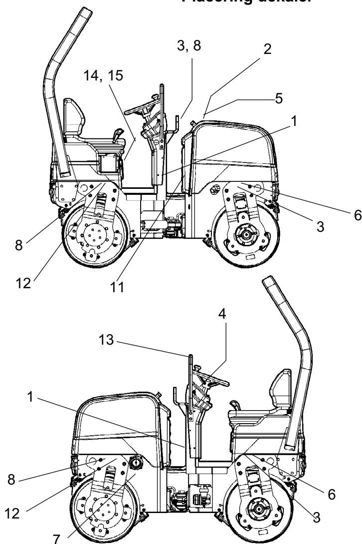
Fig. Placering, dekal och skyltar
