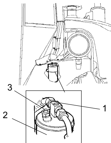
Fig. Torkfilter 1. Siktglas 2. Filterbehållare 3. Fuktdikator
