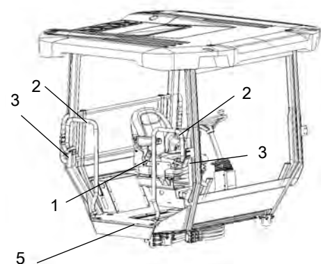
Fig. Sedile di guida 1. Cintura di sicurezza 2. Ringhiere di protezione 3. Manopola di bloccaggio 4. Protezioni antiscivolo
