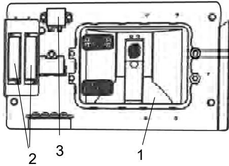
Fig. Quadro elettrico principale 1. Unità di controllo (ECU) 2. Fusibili 3. Relè principale
