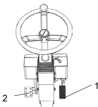
Fig. Quadro di controllo 1. Acceleratore 2. Pedale del freno
