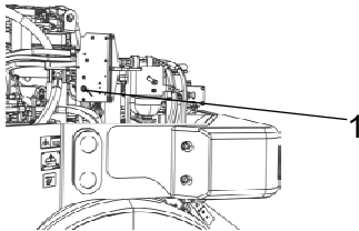
Fig. 10 Vano motore 1. Sezionatore della batteria
