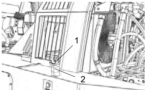
Fig. Serbatoio del carburante 1. Tappo del serbatoio 2. Tubo di rifornimento
