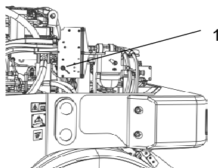
Fig. 10 Vano motore 1. Sezionatore della batteria
