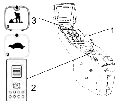
Fig. Quadro di controllo 1. Leva di comando avanti/indietro 2. Comando freno di stazionamento 3. Bassa velocità
