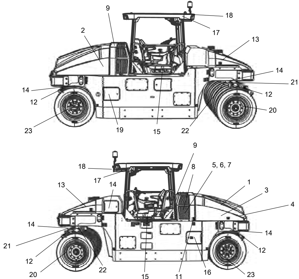
Fig. Punti di manutenzione e intervento
