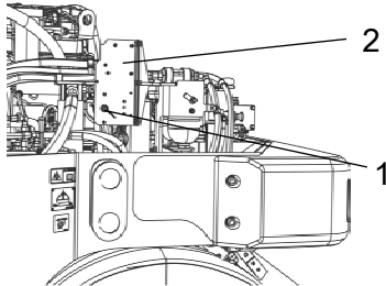
Fig. Vano batteria 1. Interruttore principale 2. Pannello fusibili principali
