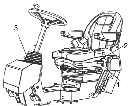
Fig. Posizione dell'operatore 1. Leva di bloccaggio per lo spostamento trasversale 2. Leva di bloccaggio per la rotazione 3. Leva di bloccaggio per l'angolo del piantone dello sterzo
