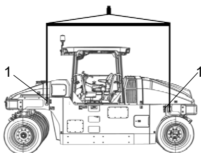
Fig. Preparazione del rullo al sollevamento 1. Targhetta per il sollevamento
