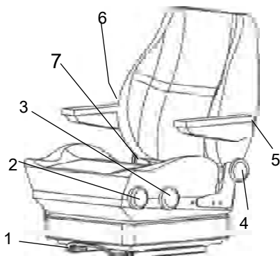
Fig. Sedile di guida 1. Leva - regolazione in senso longitudinale 2. Rotella - regolazione di altezza 3. Rotella - inclinazione del cuscino del sedile 4. Rotella - inclinazione dello schienale 5. Rotella - inclinazione dei braccioli 6. Rotella - regolazione del supporto lombare 7. Cintura di sicurezza
