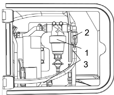
Fig. Gruppo pompa 1. Alloggiamento del filtro 2. Rubinetto 3. Raccordi rapidi
