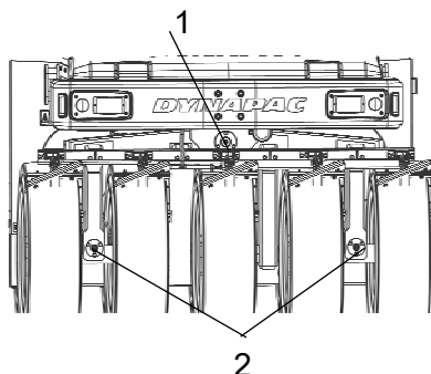
Fig. Supporto dello sterzo
