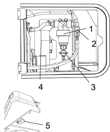
Fig. Gruppo pompa, lato destro telaio anteriore
