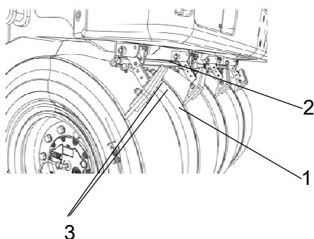
Fig. Raschietti degli pneumatici 1. Lama del raschietto 2. Gancio di bloccaggio 3. Vite di regolazione
