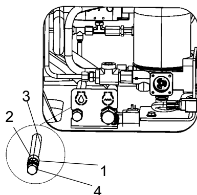
Fig. Tappi di scarico 1. Dado esagonale 2. Gomito stagno 3. Tubo flessibile 4. Tappo di scarico
