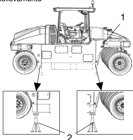
Fig. Rullo alzato con il martinetto 1. Piastra di sollevamento 2. Martinetto
