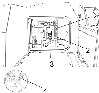
Fig. Pompa di irrorazione 1. Valvola 2. Tubo flessibile 3. Filtro grosso 4. Valvola
