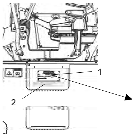
Fig. Piattaforma di guida 1. Targhetta di identificazione della macchina 2. Targhetta di identificazione del motore
