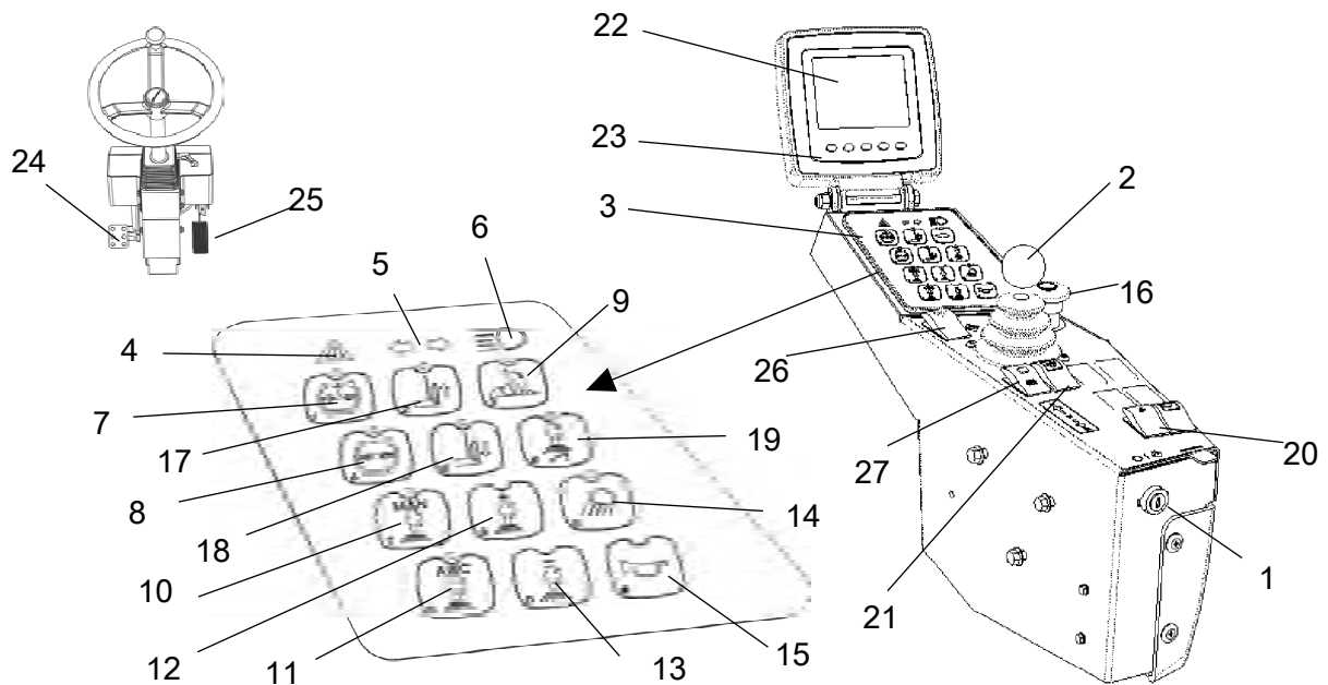
Fig. Quadro di controllo
