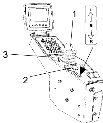
Fig. Quadro di comando 1. Leva di comando avanti/indietro 2. Freno di parcheggio 3. Prova freni
