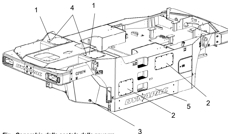
Fig. Coperchio della scatola della zavorra
