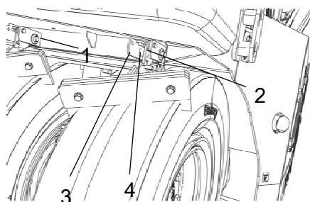
Fig. Raschietti 1. Spina 2. Forcella 3. Gancio di bloccaggio 4. Raschietto
