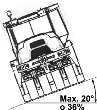
Fig. Funzionamento su pendenze
