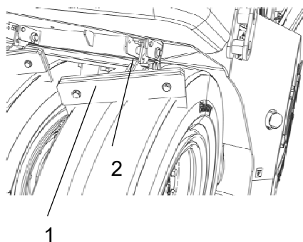
Fig. Raschietti degli pneumatici 1. Lama del raschietto 2. Gancio di bloccaggio
