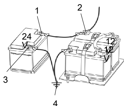
Fig. Avviamento di emergenza
