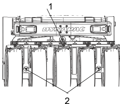
Fig. Supporto dello sterzo 1. Ingrassatore x 1 Supporto dello sterzo superiore 2. Ingrassatore x 2 Supporto dello sterzo inferiore
