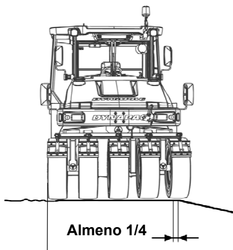
Fig. Posizione delle ruote durante la guida su bordi
