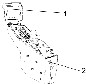
Fig. Quadro di comando 1. Display 2. Chiave di accensione
