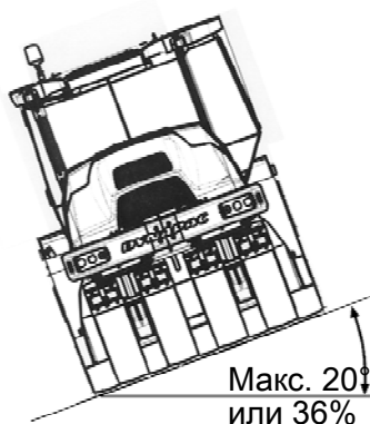
Рис. Работа на откосах
