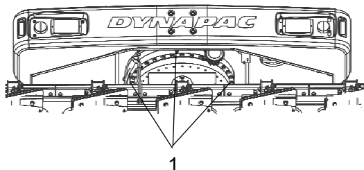
Рис. Поворотный подшипник 1. Ниппели для смазки (4 шт.)
