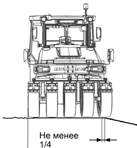
Рис. Расположение колёс при движении по краю
