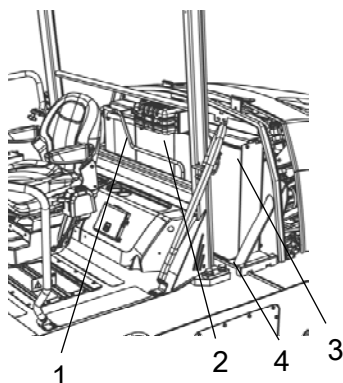
Рисунок. Радиатор
