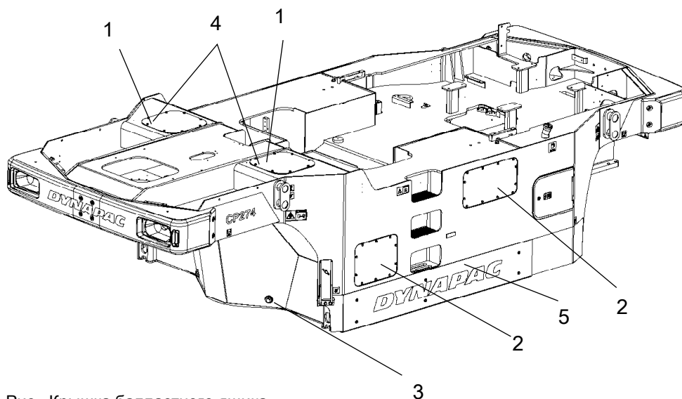
Рис. Крышка балластного ящика
