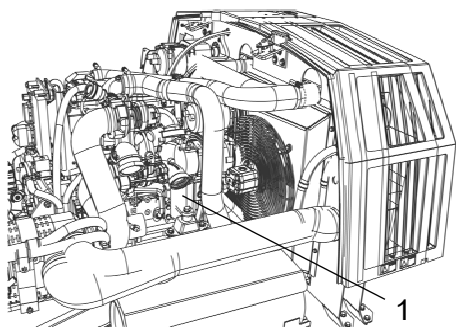
Рис. Моторный отсек 1. Масляный фильтр
