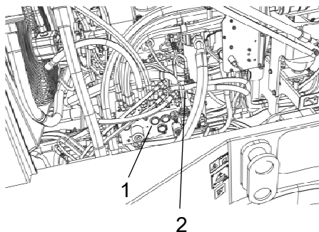
Рис. Клапан растормаживания
