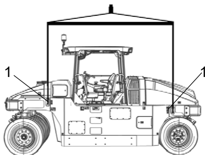
Рис. Подготовленный к подъёму каток 1. Табличка
