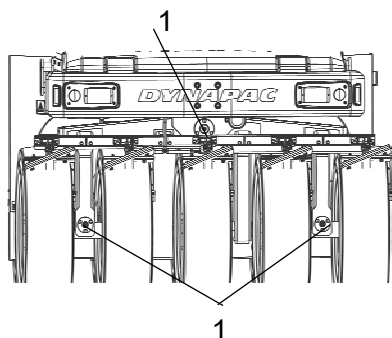
Рис. Поворотный подшипник 1. Смазочный ниппель (1 шт.), верхний поворотный подшипник 2. Смазочные ниппели (2 шт.), нижний поворотный подшипник
