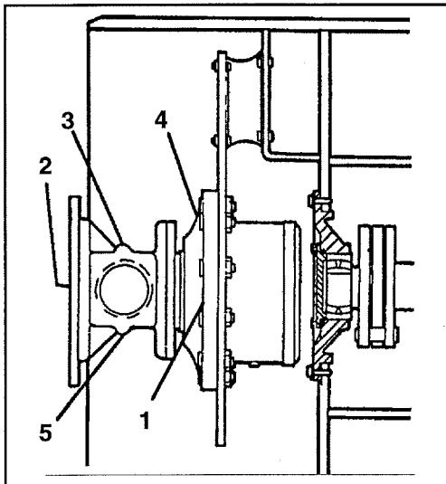
Abb. 39 Bandagengetriebe 1 Füllstandschaube 2 Füllstandschaube 3 Einfüllschraube 4 Einfüllschraube 5 Ablaßschraube
