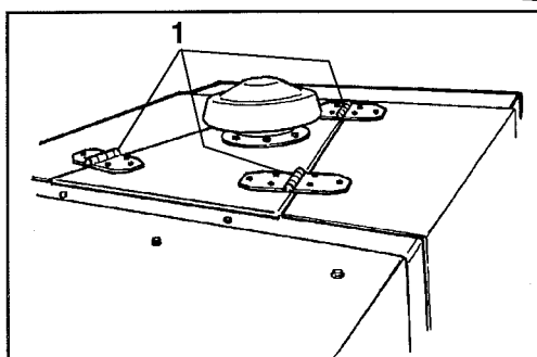
Abb. 28 Motorhaube 2 Scharnier
