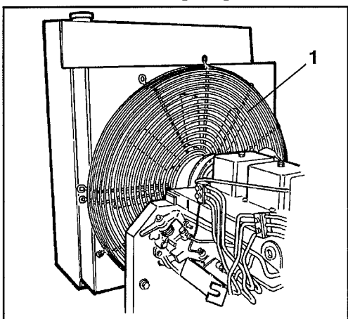
Abb. 27 Motorraum 1 Hydraulikölkühler
