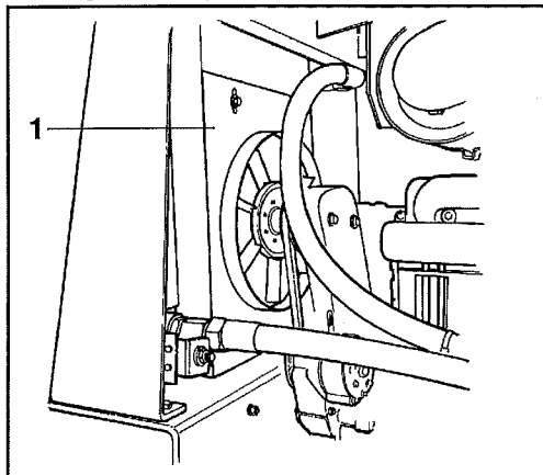
Abb. 26 Motorraum 1 Hydraulikölkühler
