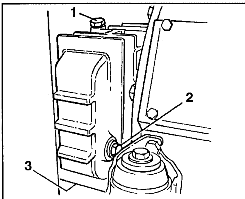
Abb. 37 Verteilergetriebe, linke Seite 1 Einfüllschraube 2 Meßschraube 3 Ablassschraube
