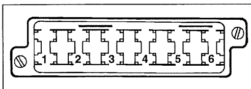
Abb. 43 Sicherungsdose im Kabinendach
