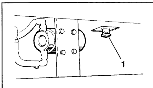
Abb. 40 Wassertank 1 Ablaßhahn
