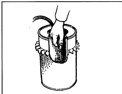
Abb. 12 Filterpatrone
