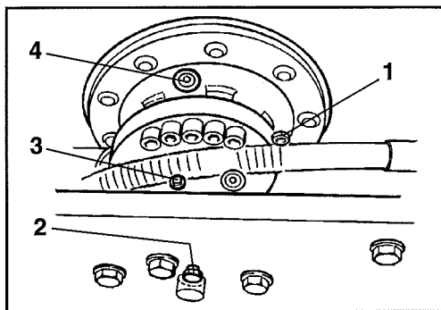
Abb. 30 Bandagengetriebe 1 Füllstandschaube 2 Füllstandschaube 3 Einfüllschaube 4 Einfüllschaube
