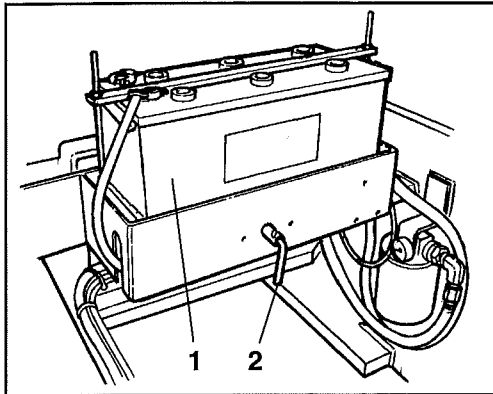
Abb. 14 Batteriefach 1 Batterie 2 Batterietrennschalter
