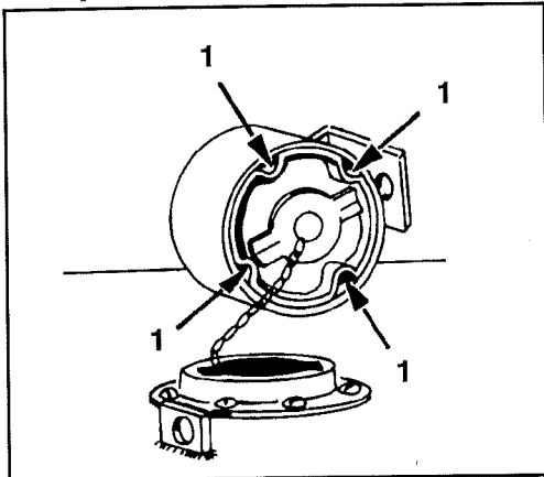
Abb. 20 Tankdeckel 1 Luftloch
