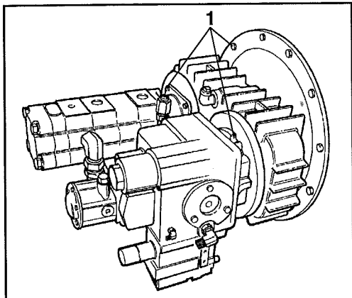
Abb. 23 Hydraulikpumpen 1 Pumpenbefestigung
