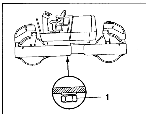
Abb. 33 Linke Seite der Walze 1 Ablaßschraube
