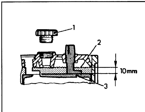
Abb. 15 Flüssigkeitsstand in der Batterie 1 Verschlusskappe 2 Flüssigkeitsstand 3 Platte
