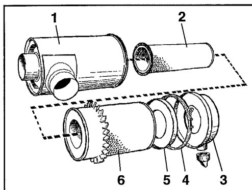
Abb. 34 Luftfilter 1 Filtergehäuse 2 Sicherheitspatrone 3 Deckel 4 Klammer 5 Innendeckel 6 Filterpatrone
