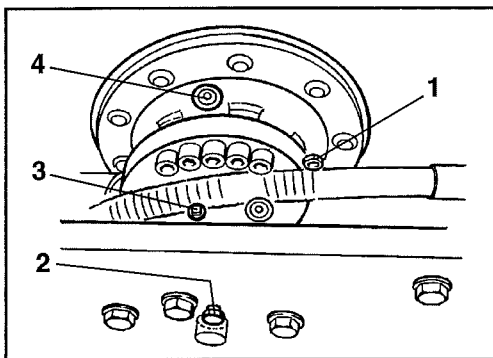
Abb. 38 Bandagengetriebe 1 Füllstandschaube 2 Füllstandschaube 3 Einfüllschraube 4 Einfüllschraube
