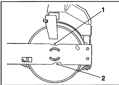
Abb. 36 Bandage, rechte Seite 1 Ablass-/Einfüllöffnung 2 Schauglas
