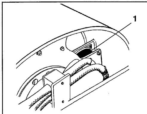
Abb. 16 Bandagenaufhängung 1 Gummierelemente
