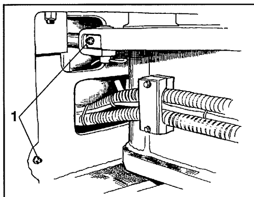
Abb. 19 Lenkgelenk/linke Seite 1 Schmiernippel
