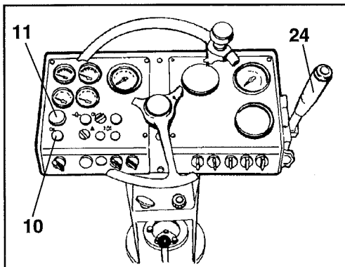
Abb. 4 Armaturenbrett 10 Bremswarnleuchte 11 Notstoptaste 24 Vorwärts-/Rückwärtsfahrhebel
