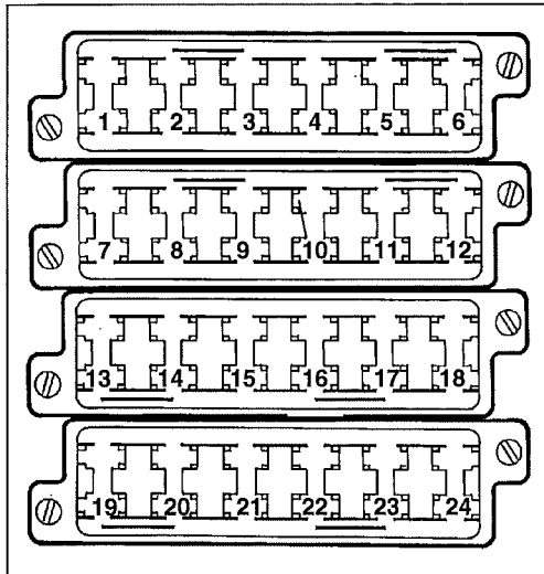
Abb. 42 Sicherungsdose
