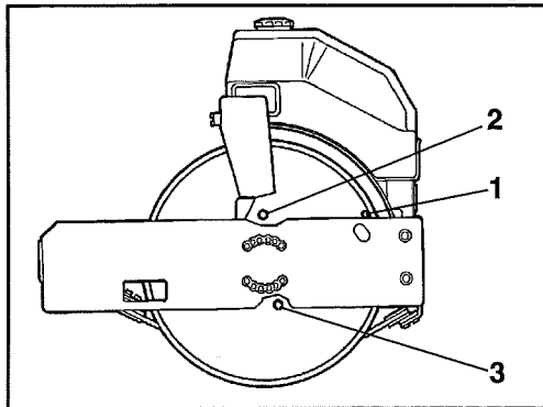
Abb. 29 Rechte Bandageseite 1 Ölmeßstab 2 Einfüllstutzen 3 Schauglas
