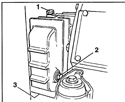
Abb. 31 Verteilergetriebe, linke Seite 1 Einfüllschaube 2 Meßschaube 3 Abflaßschaube
