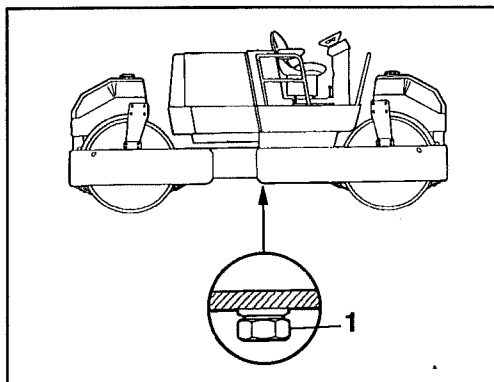
Abb. 32 Rechte Seite der Walze 1 Ablaßhahn
