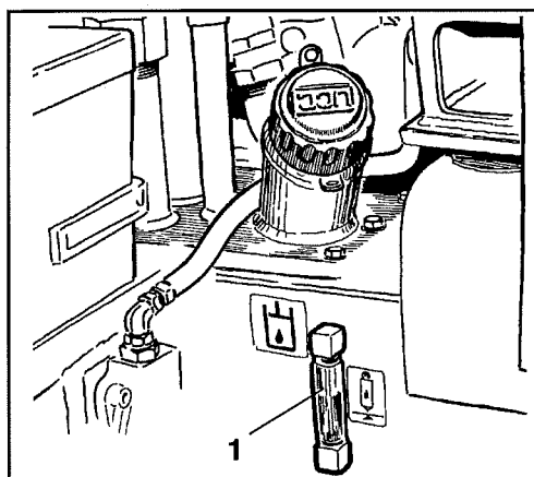
Fig. 6 Serbatoio olio idraulico 1 Vetro di ispezione
