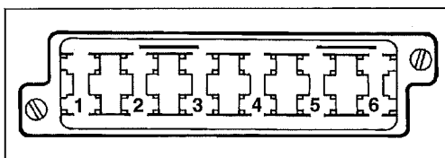
Fig. 43 Scatola fusibili in cabina
