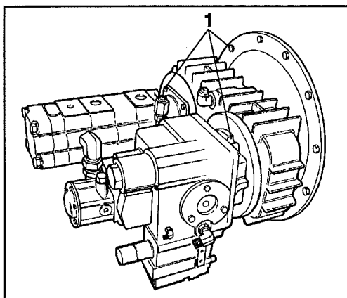
Fig. 23 Pompe idrauliche 1 Fissaggi pompe
