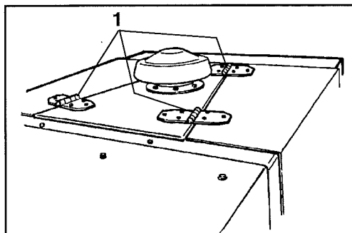
Fig. 28 Cafano motore 1 Cerniera
