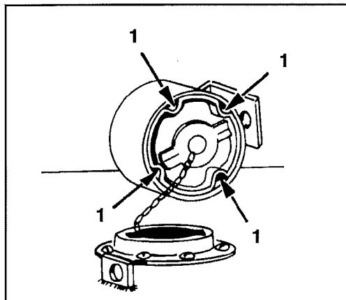
Fig. 20 Tappo serbatoio 1 Foro di aerazione
