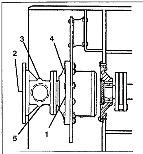
Fig. 39 Scatola riduttore vista di lato
