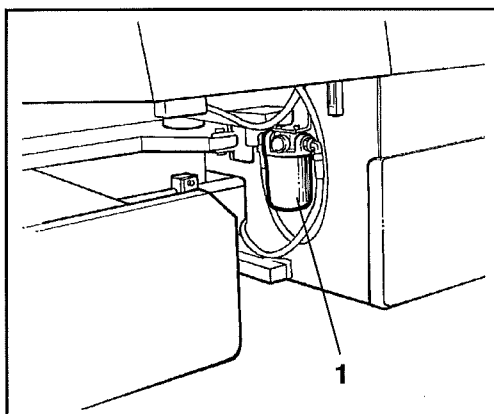
Fig. 24 Lato destro allo snodo dello sterzo 1 Filtro di ritorno - impianto sterzo
