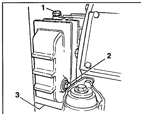
Fig. 37 Scatola di rinvio, lato sinistro 1 Tappo di rifornimento 2 Tappo di livello 3 Tappo di scarico
