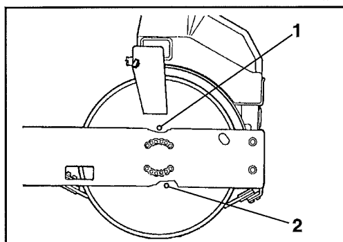
Fig. 36 Rullo, lato destro 1 Tappo di scarico/rifornimento 2 Tappo di livello
