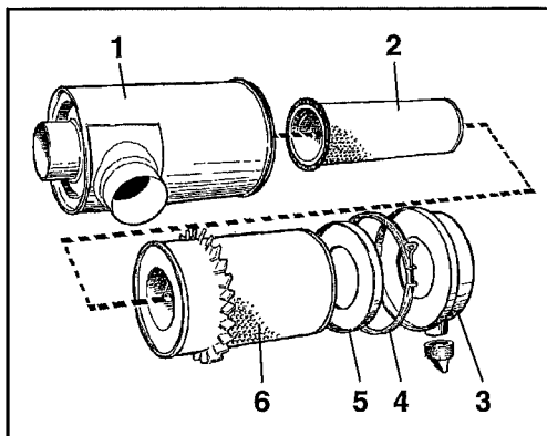
Fig. 11 Depuratore aria
