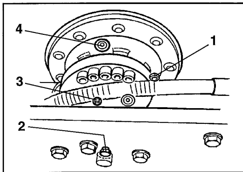
Fig. 38 Scatola riduttore
