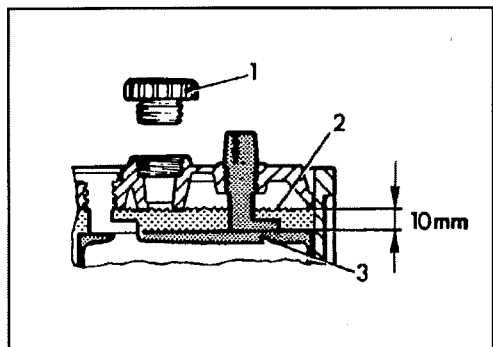
Fig. 15 Livello dell'elettrolita nella batteria
