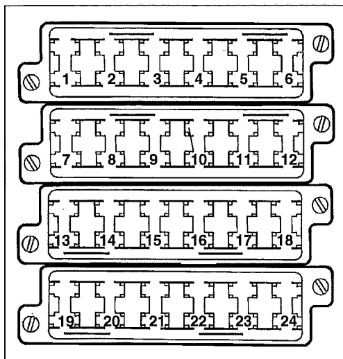
Fig. 42 Scatole dei fusibili
