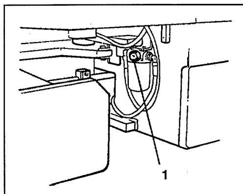
Fig. 21 Lato sinistro allo snodo dello sterzo 1 Indicatore del filtro
