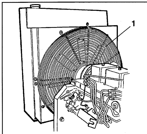
Fig. 27 Vano motore 1 Radiatore olio idraulico
