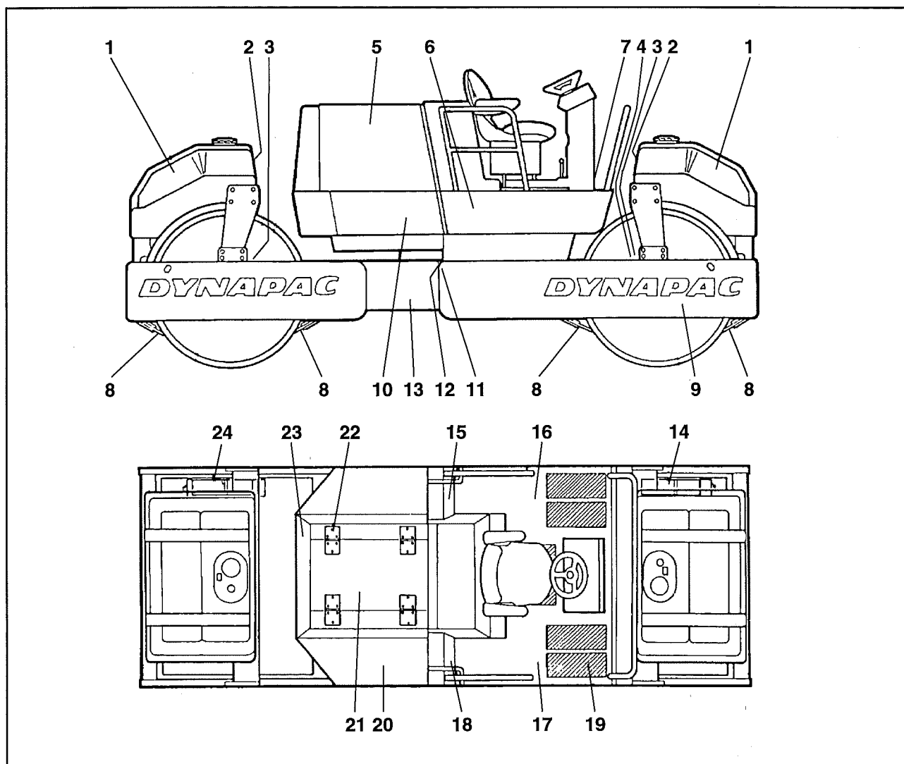
Fig. 1 Punti di intervento
