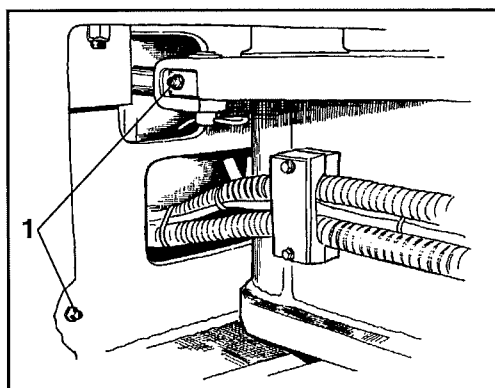
Fig. 19 Snodo sterzo/lato sinistro 1 Nippli di ingrassaggio
