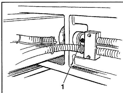
Fig. 18 Inclinatore/lato destro 1 Nippli di ingrassaggio
