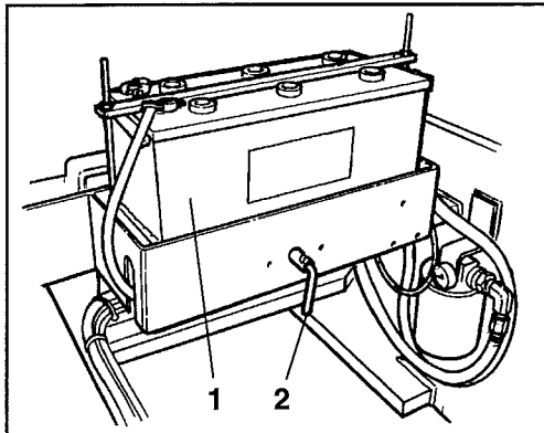
Fig. 14 Sede della batteria
