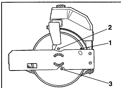
Fig. 29 Lato destro rullo 1 Astina di livello 2 Rifornimento 3 Vetro di ispezione
