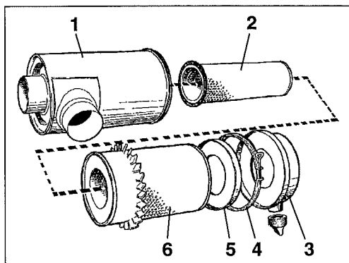
Fig. 34 Depuratore aria 1 Depuratore 2 Filtro di sicurezza 3 Coperchio esterno/raccoglitore polvere 4 Fascetta 5 Coperchio interno 6 Filtro principale
