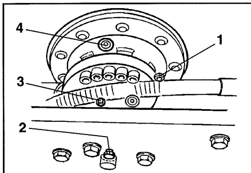
Fig. 30 Scatola riduttore 1 Tappo di livello 2 Tappo di livello 3 Tappo di rifornimento 4 Tappo di rifornimento
