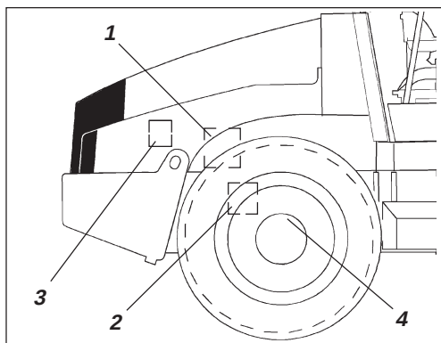
Afb. 25 Rechter machinekant
