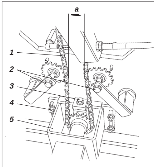
Afb. 33 Onderkant van de chauffeursplaats
