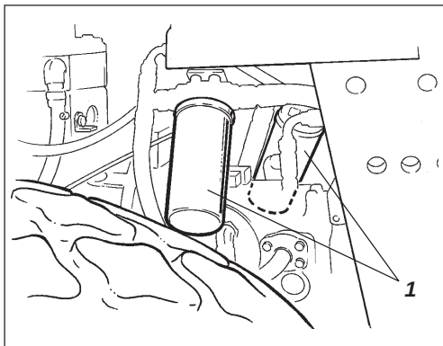
Afb. 36 Motorruimte 1. Hydraulische olie-filter (2)
