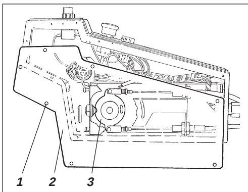
Afb. 46 Vooruit-/achteruithendel
