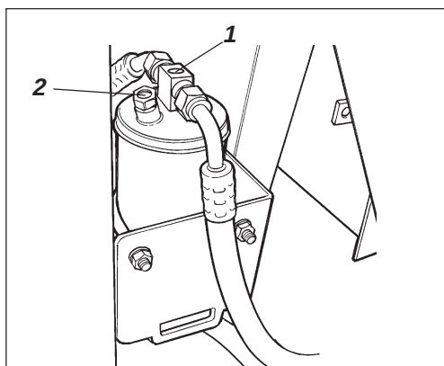
Afb. 51 Droogfilter in de motorruimte
