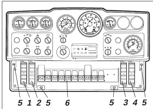
Afb. 53 Instrumentenpaneel
