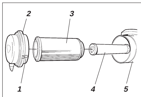
Afb. 11 Luchtfilter
