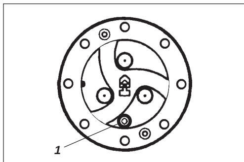
Afb. 41 Planeetoverbrenging/aftappositie 1. Plug
