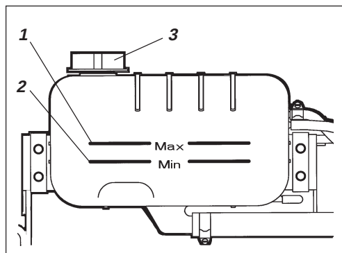
Afb. 6 Radiator 1. Max. peil 2. Min. peil 3. Bijvuldop
