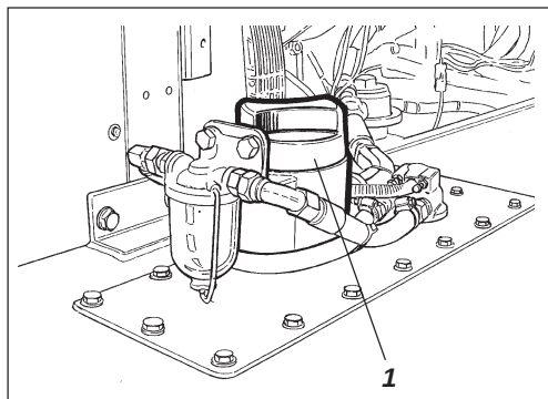
Afb. 8 Brandstoftank 1. Bijvulpijp
