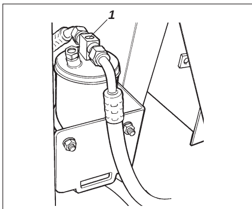
Afb. 18 Droogfilter 1. Kijkglas
