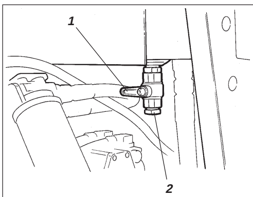
Afb. 37 Onderzijde hydraulische tank 1. Aftapkraan 2. Plug
