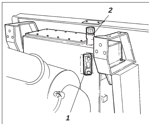
Afb. 9 Hydraulische olietank 1. Peilglas 2. Bijvulpijp
