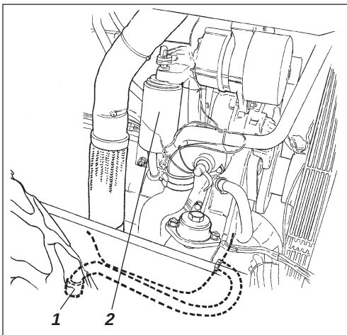
Afb. 32 Linker motorzijde 1. Aftapplug 2. Oliefilter
