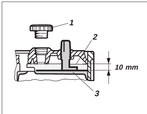
Afb. 28 Vloeistofpeil in accu
