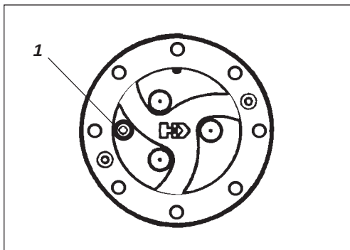
Afb. 22 Niveaucontrole – planeetoverbrenging 1 Niveau/Bijvulplug
