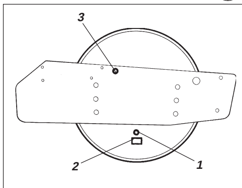
Afb. 45 Wals, rechterkant 1. Aftap/bijvulplug 2. Nummerplaat 3. Peilglas
