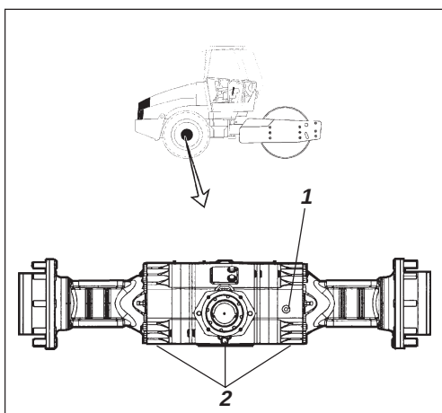
Afb. 40 Achteras 1. Niveau/bijvulplug 2. Aftappluggen
