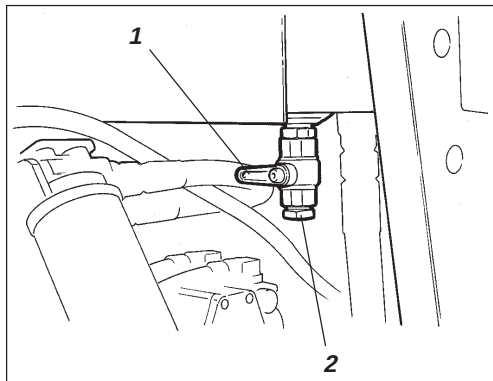
Afb. 44 Hydraulische tank, onderkant 1. Afsluitkraan 2. Plug
