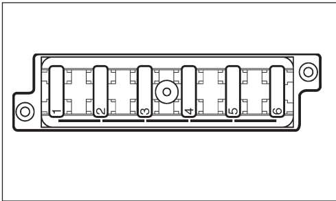
Afb. 55 Zekeringenkast in cabinedak
