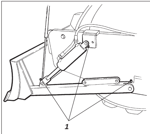
Afb. 20 Egaliseerblad 1. Smeernippels
