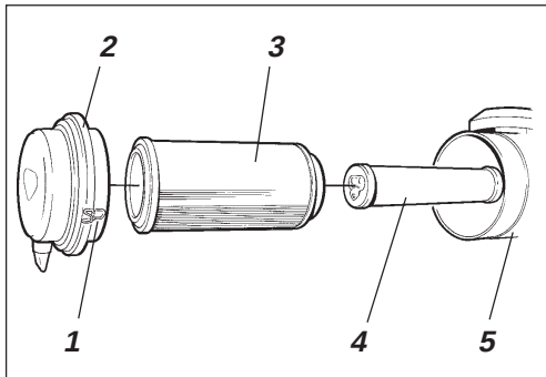
Afb. 39 Luchtfilter 1. Vergrendelkleppen 2. Deksel 3. Hoofdfilter 4. Veiligheidsfilter 5. Filterhuis
