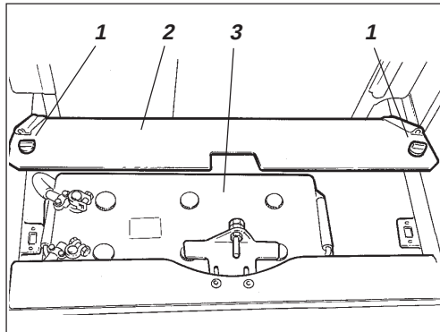
Afb. 27 Accubak
