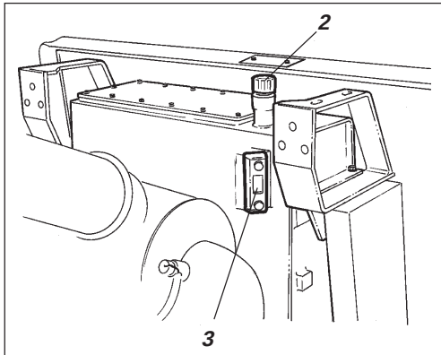
Afb. 35 Tank hydraulische olie 2. Bijvuldop/Ontluchttingsfilter 3. Peilglas
