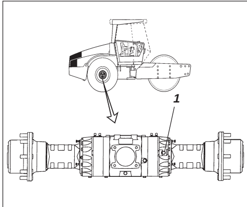
Afb. 21 Niveaucontrole – differentieelhuis 1 Niveau/Bijvulplug
