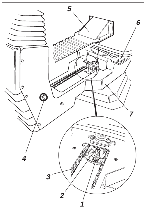
Afb. 34 Stoellager
