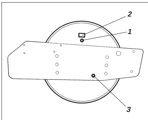
Afb. 23 Rechterkant van de wals 1. Bijvuldop 2. Nummerplaat 3. Peilglas
