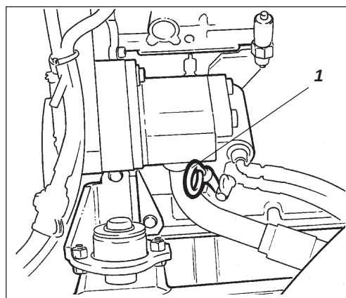
Afb. 7 Motorruimte 1. Oliepeilstok
