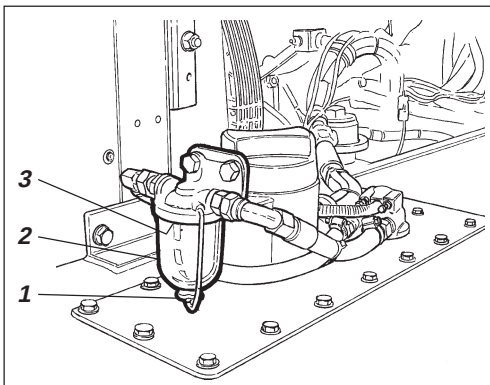
Afb. 31 Motor 1. Schroef 2. Glasreservoir 3. Zeef
