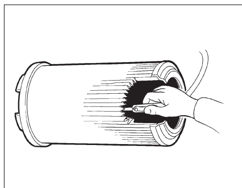
Afb. 12 Hoofdfilter
