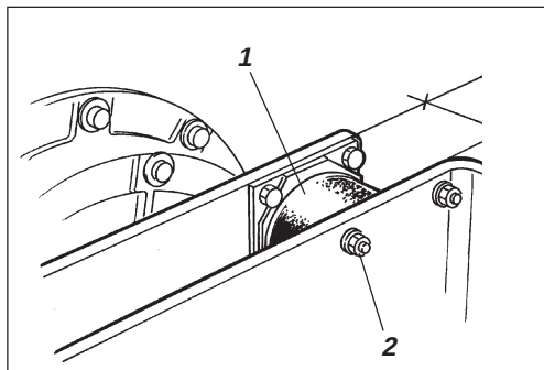
Afb. 26 Wals trillingkant
