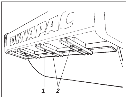
Fig. 3 Skraper 1. Skrapeblad 2. Skruer
