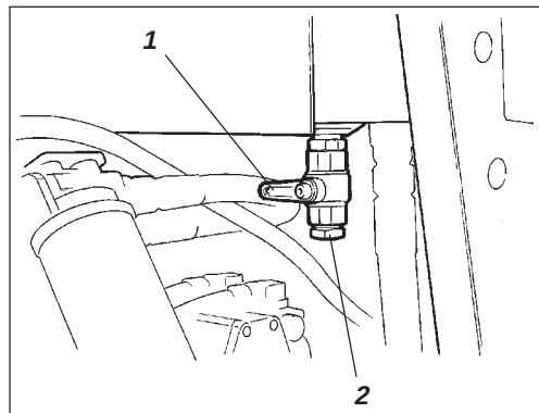
Fig. 50 Hydraulikk tank, underside
