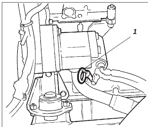
Fig. 8 Motorrom 1. Peilepinne for oljemåling
