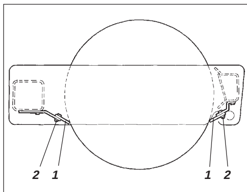
Fig. 5 Skraper
