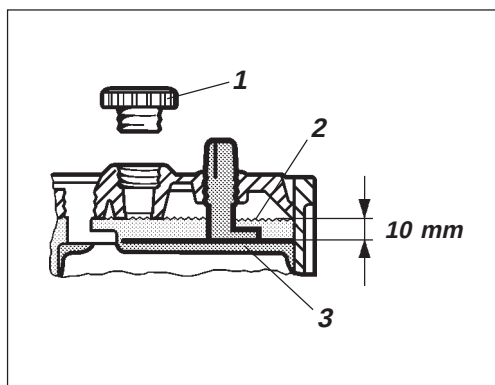
Fig. 34 Væsknivå i batteri
