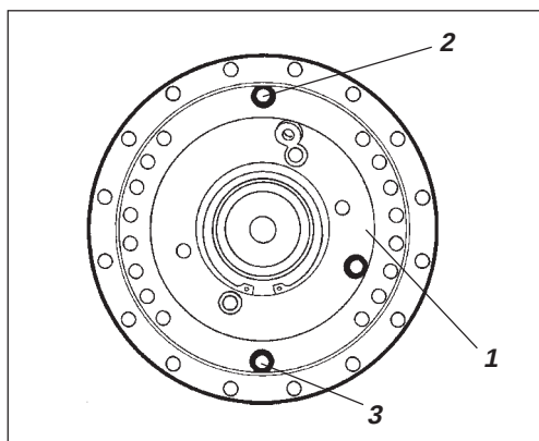
Fig. 25 Nivåkontroll – valsgirkasse
