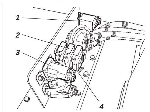
Fig. 64 Motorrom
