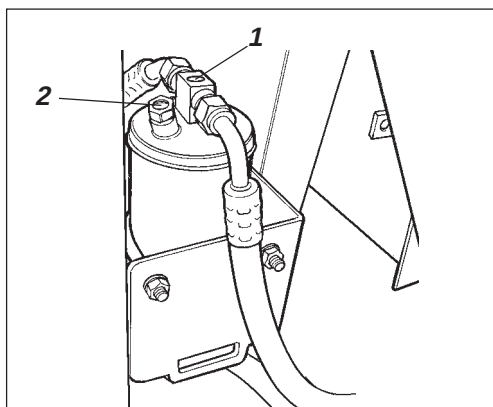
Fig. 59 Tørkefilter i motorrom
