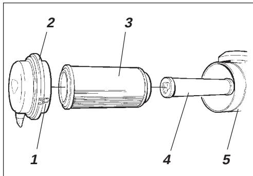
Fig. 12 Luftrenser
