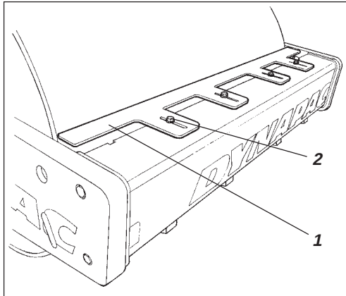
Fig. 2 Skraper 1. Skrapeblad 2. Skruer (x4)
