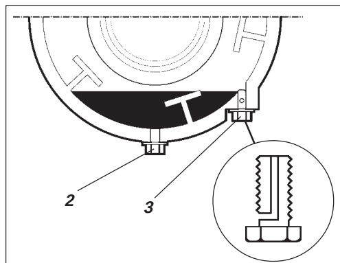
Fig. 28 Valkassett 2. Tappeplugg 3. Nivårør
