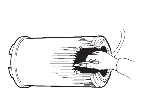
Fig. 13 Hovedfilter
