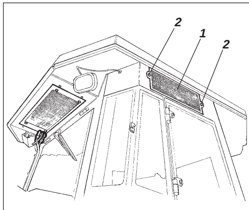
Fig. 49 Førerhus 1. Friskluftfilter 2. Skruv (x2)
