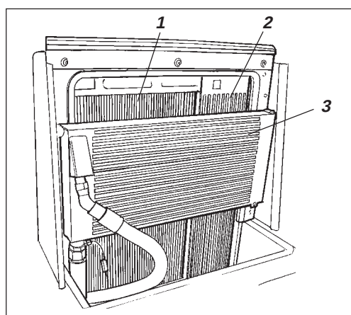
Fig. 30 Motorrom 1. Vannkjøler 2. Ladeluftkjøler 3. Hydraulikkoljekjøler
