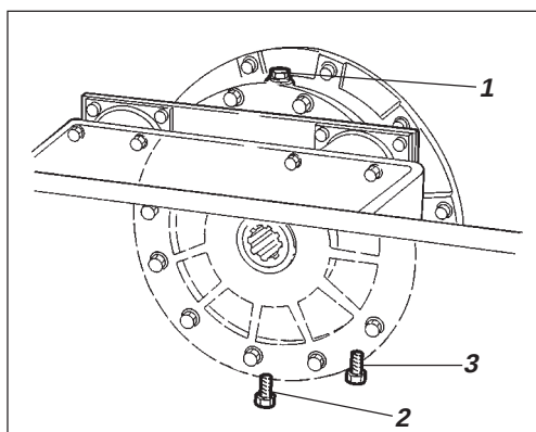
Fig. 27 Høyre valsside
