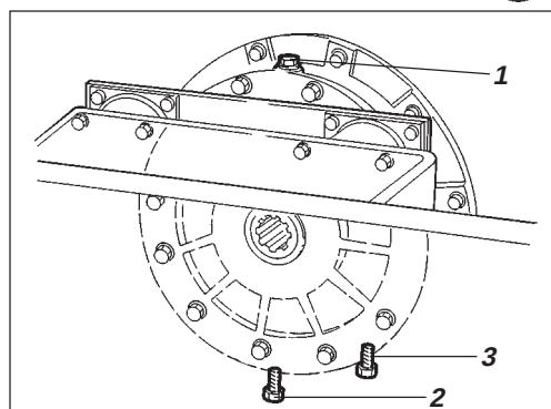
Fig. 52 Vals, høyre side
