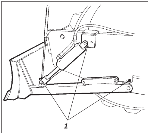
Fig. 21 Avjevnerblad 1. Smørenipler
