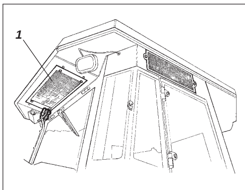
Fig. 20 Førerhus
