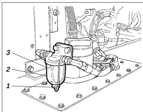
Fig. 37 Motor 1. Skruer 2. Glassbeholder 3. Sil
