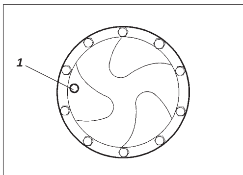
Fig. 23 Nivåkontroll – planetgir (CA 262-362 Std.) 1. Nivå-/påfyllingsplugg
