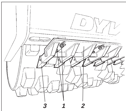
Fig. 4 Skraper 1. Skruer 2. Skrapebjelke 3. Skrapetennene
