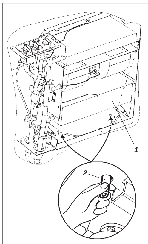
Fig. 57 Luftkondisjonering 1. Kjøleelement 2. Dreneringsventil (x2)
