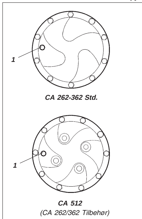
Fig. 48 Planetgir/stilling for påfylling 1. Plugg
