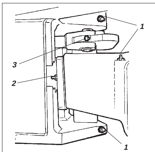
Fig. 16 Styreledd høyre side
