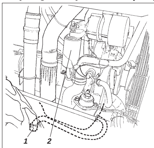
Fig. 38 Venstre motorside 1. Tappeplugg 2. Oljefilter
