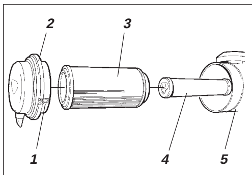
Fig. 45 Luftrenser 1. Låseklaffer 2. Lokk 3. Hovedfilter 4. Sikkerhetsfilter 5. Filterhus
