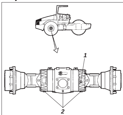
Fig. 46 Bakaksel 1. Nivå-/påfyllingsplugg 2. Avtappingsplugg
