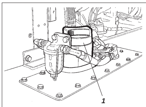
Fig. 9 Drivstofftank 1. Påfyllingsrør
