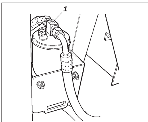
Fig. 19 Tørkefilter
