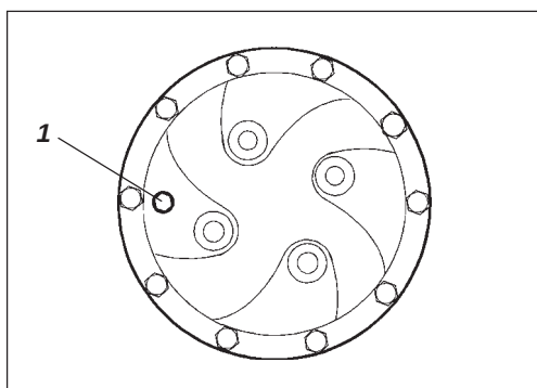
Fig. 24 Nivåkontroll – planetgir (CA 512 std) (CA 262-362 tilbehør) 1. Nivå-/påfyllingsplugg
