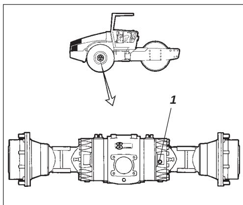
Fig. 22 Nivåkontroll – differensialhus 1. Nivå-/påfyllingsplugg
