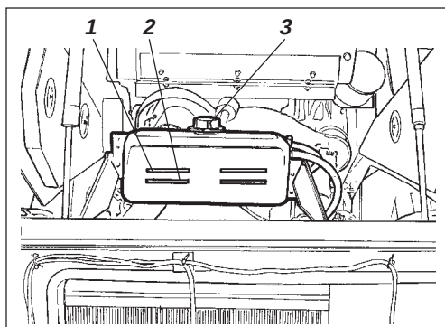
Fig. 7 Kjøler
