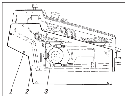
Fig. 54 Forover-/bakoverspak
