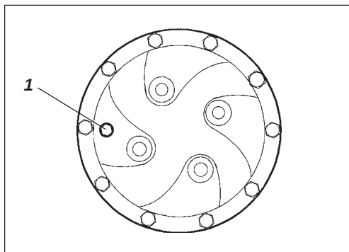
Fig. 20 Nivåkontroll - planetväxel, tillbehör 1. Nivå-/Påfyllningsplugg
