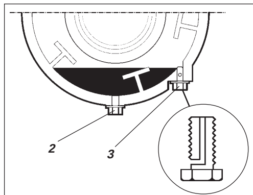
Fig. 24 Valkassett 2. Avtappningsplugg 3. Nivåplugg
