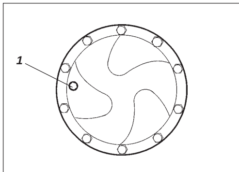
Fig. 19 Nivåkontroll - planetväxel, std 1. Nivå-/Påfyllningsplugg
