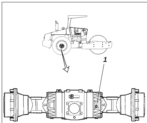
Fig. 18 Nivåkontroll - differentialhus 1. Nivå-/Påfyllningsplugg
