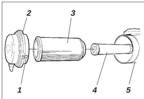
Fig. 37 Luftrenare
