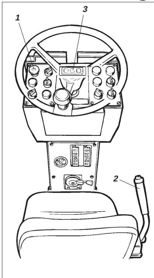
Fig. 10 Reglagepanel
