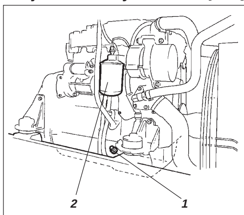
Fig. 32 Vänster motorsida 1. Avtappningsplugg 2. Oljefilter
