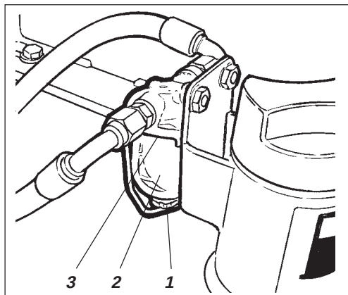
Fig. 31 Motor 1. Mutter 2. Glas behållare 3. Sil
