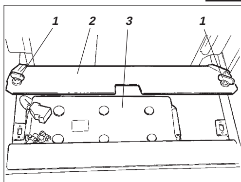
Fig. 29 Batterilåda
