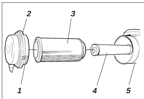
Fig. 36 Depurador de aire
