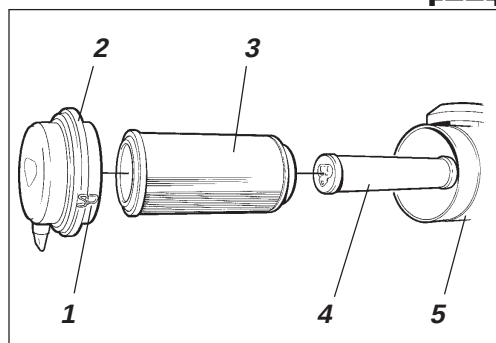
Fig. 11 Depurador de aire
