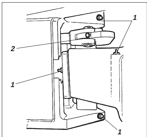
Fig. 15 Articulación de dirección, lateral derecho
