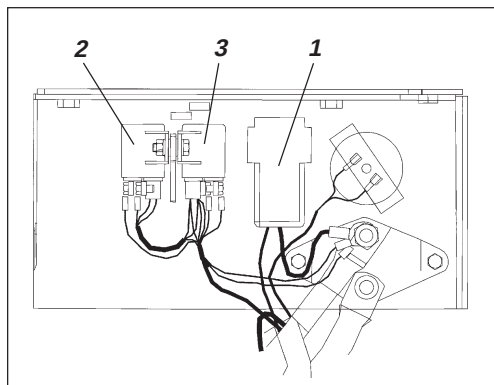
Fig. 51 Compartimento del motor
