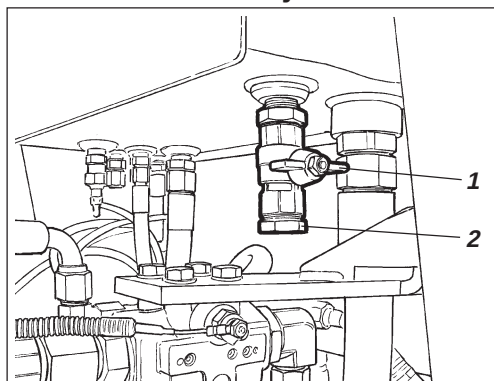
Fig. 34 Parte inferior del depósito hidráulico
