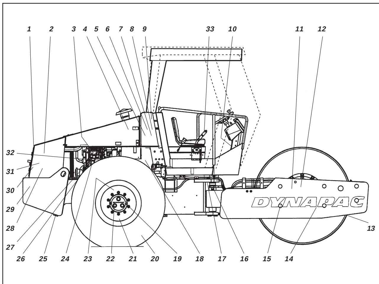
Fig.1 Puntos de servicio
