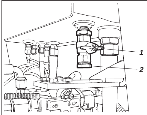
Fig. 40 Depósito de líquido hidráulico, bajos
