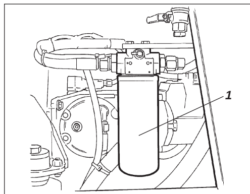
Fig. 33 Alojamiento del motor 1. Filtro de aceite hidráulico (x1)
