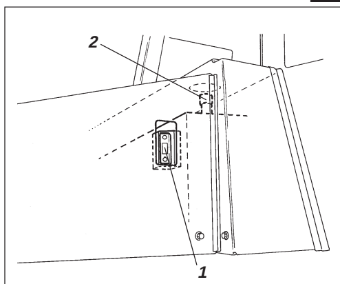
Fig. 9 Depósito de líquido hidráulico 1. Mirilla de nivel 2. Tubo de llenado
