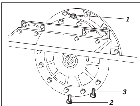
Fig. 42 Rodillo, lado derecho 1. Tapón de llenado 2. Tapón de vaciado 3. Tapón de nivel
