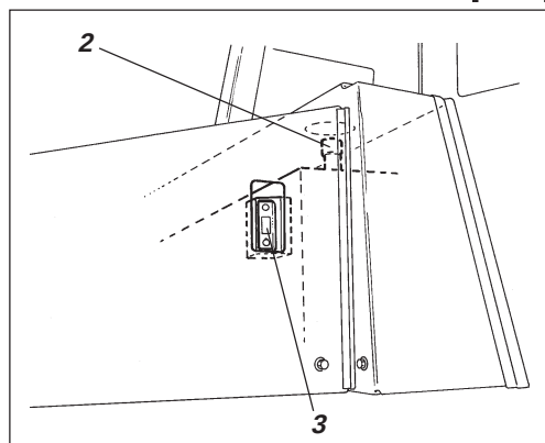
Fig. 32 Depósito de líquido hidráulico 2. Tapa de llenado/Filtro de aire 3. Mirilla de nivel
