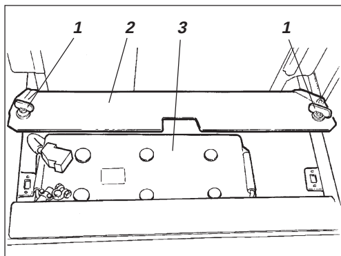
Fig. 29 Caja de la batería 1. Tornillos rápidos 2. Alojamiento de la batería 3. Batería
