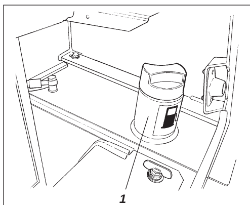
Fig. 8 Depósito de combustible 1. Tubo de llenado
