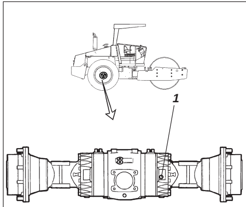
Fig. 18 Control de nivel – alojamiento del diferencial
