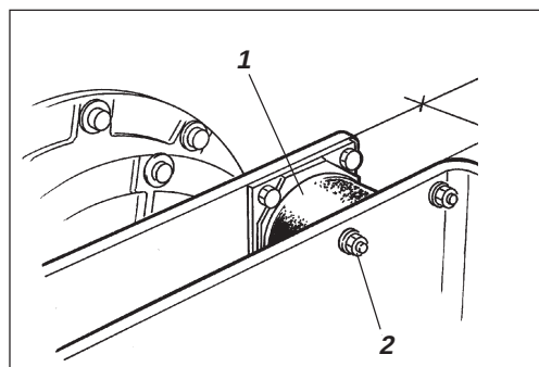
Fig. 28 Lado vibrante del rodillo 1. Pieza de goma 2. Tornillos de sujeción
