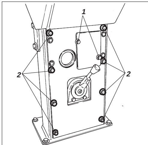
Fig. 47 Panel de instrumentos
