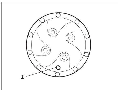
Fig. 38 Engranaje planetario / situación de vaciado
