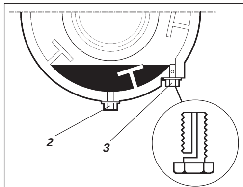
Fig. 24 Cassette de rodillo 2. Tapón de vaciado 3. Tubo de nivel
