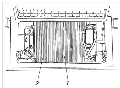
Fig. 26 Enfriador del aceite hidráulico 1. Enfriador de agua 2. Enfriador del aceite hidráulico
