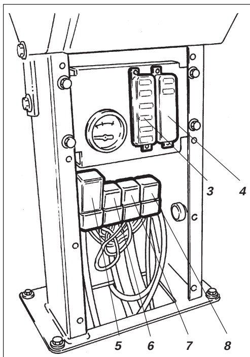
Fig. 48 Panel de instrumentos
