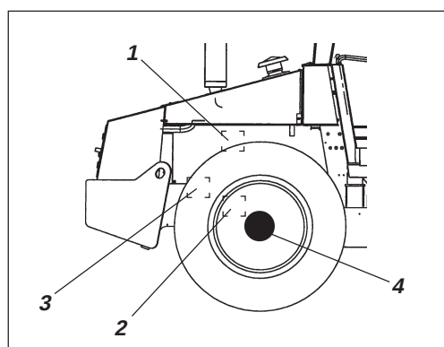
Fig. 27 Lateral derecho de la máquina 1. Bomba de dirección 2. Puente trasero 3. Suspensión del motor 4. Tuercas de ruedas
