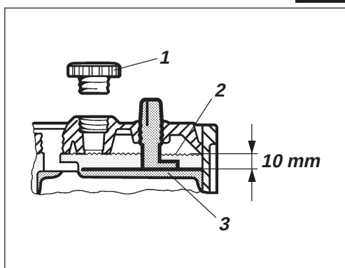
Fig. 30 Nivel de electrolito en la batería 1. Tapón de célula 2. Nivel de electrolito 3. Placa
