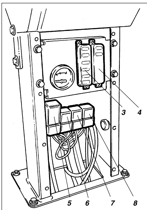
Fig. 48 Painel de instrumentos
