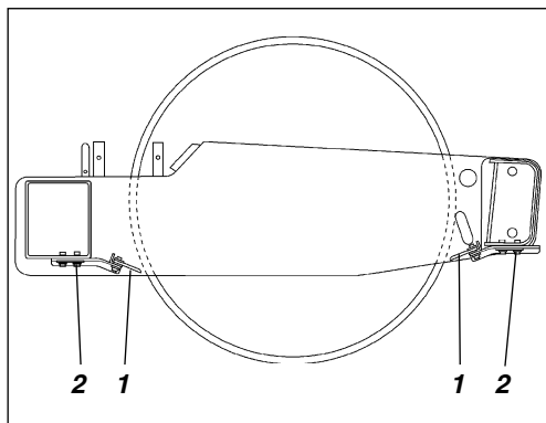
Fig. 4 Raspadeiras
