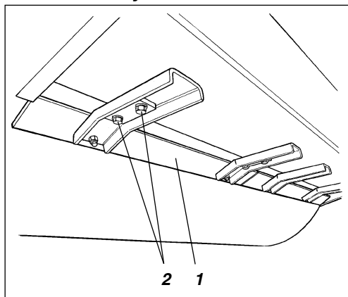
Fig. 2 Raspadeiras
