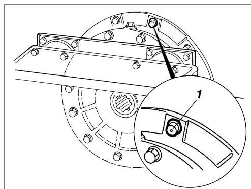
Fig. 25 Rolo 1. Parafuso com respiro
