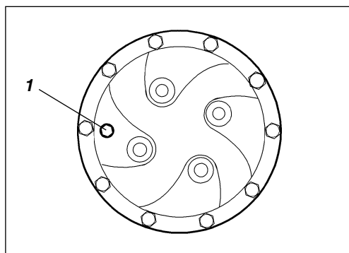
Fig. 19 Verificação de nível – cubo planetário, std
