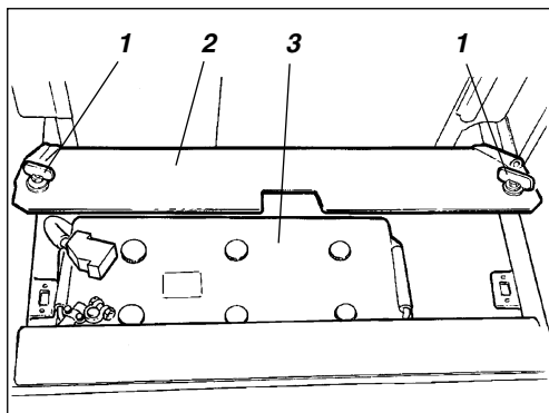
Fig. 29 Caixa da bateria 1. Parafusos rápidos 2. Tampa da bateria 3. Bateria
