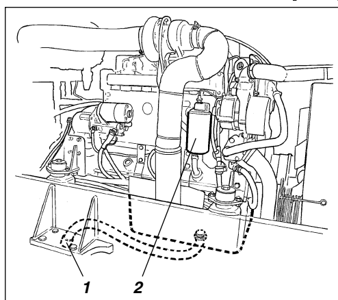
Fig. 20 Lado esquerdo do motor
