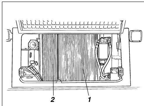
Fig. 26 Radiador do óleo hidráulico
