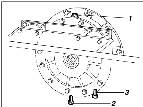
Fig. 42 Rolo, lado direito 1. Bujão de enchimento 2. Bujão de drenagem 3. Bujão de nível
