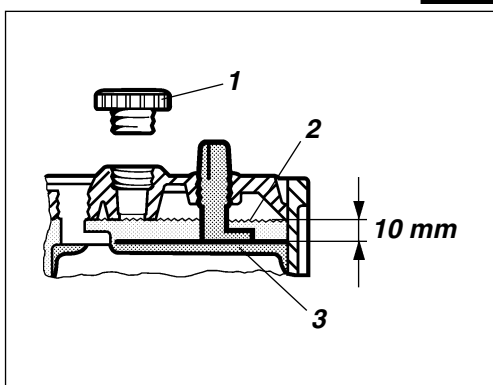
Fig. 30 Nível de electrólito na bateria 1. Tampa de elemento 2. Nível de electrólito 3. Placa
