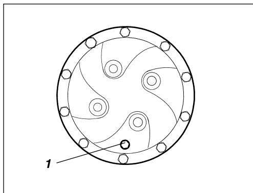
Fig. 38 Engrenagem planetária / posição de drenagem 1. Bujão
