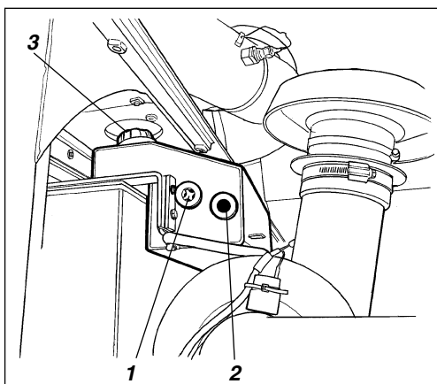
Fig. 6 Radiador
