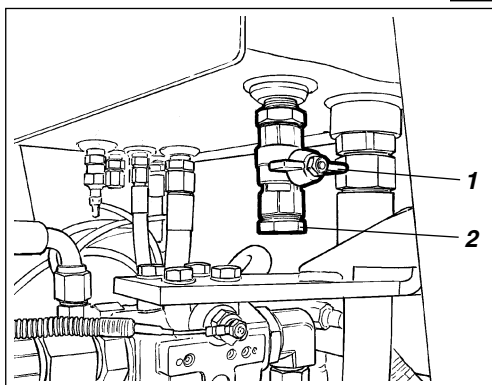
Fig. 40 Depósito hidráulico, face inferior 1. Torneira de fechamento 2. Bujão
