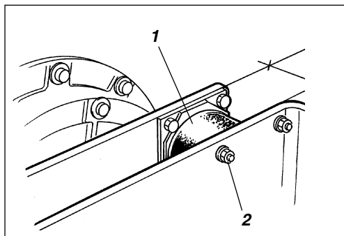
Fig. 28 Rolo, lado da vibração
