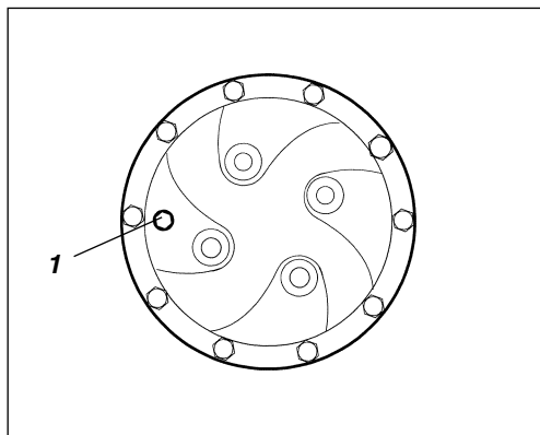
Fig. 39 Engrenagem planetária / posição de enchimento 1. Bujão
