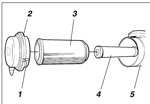
Fig. 36 Filtro do ar
