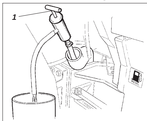
Afb. 44 Brandstoftank 1. Oliedrain pomp
