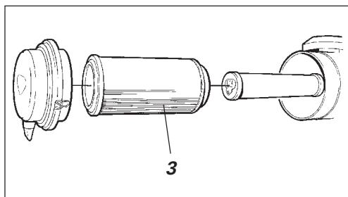
Afb. 38 Luchtfilter
