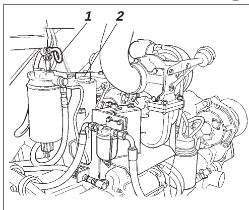
Afb. 2 Motorruimte 1. Oliepeilstok 2. Bijvuldop
