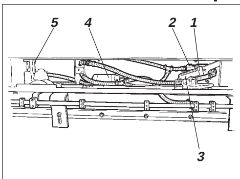
Afb. 9 Pompsysteem
