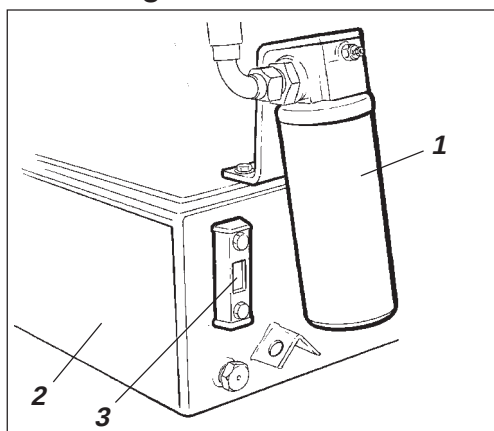
Afb. 37 Hydraulische tank
