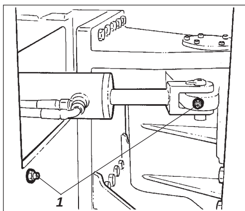
Afb. 15 Linkerzijde van de stuurverbinding 1. Smeernippels
