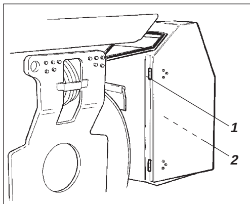
Afb. 33 Motorruimte 1. Scharnier 2. Hendelkabels
