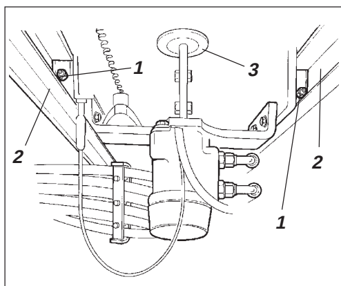
Afb. 34 Stoellager, onderkant 1. Smeernippels 2. Glijrails 3. Smeernippel
