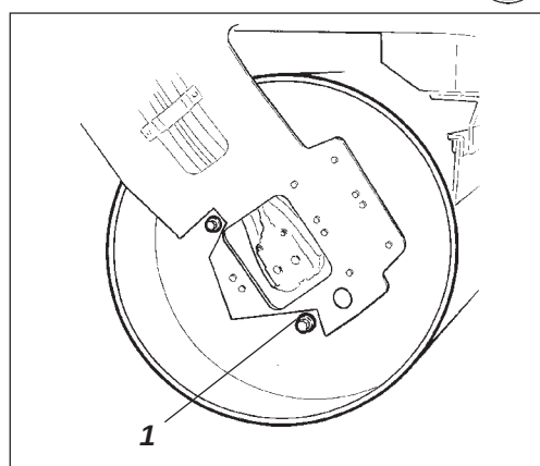
Afb. 43 Wals trillingkant 1. Aftapplug
