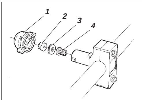
Afb. 8 Sproeier
