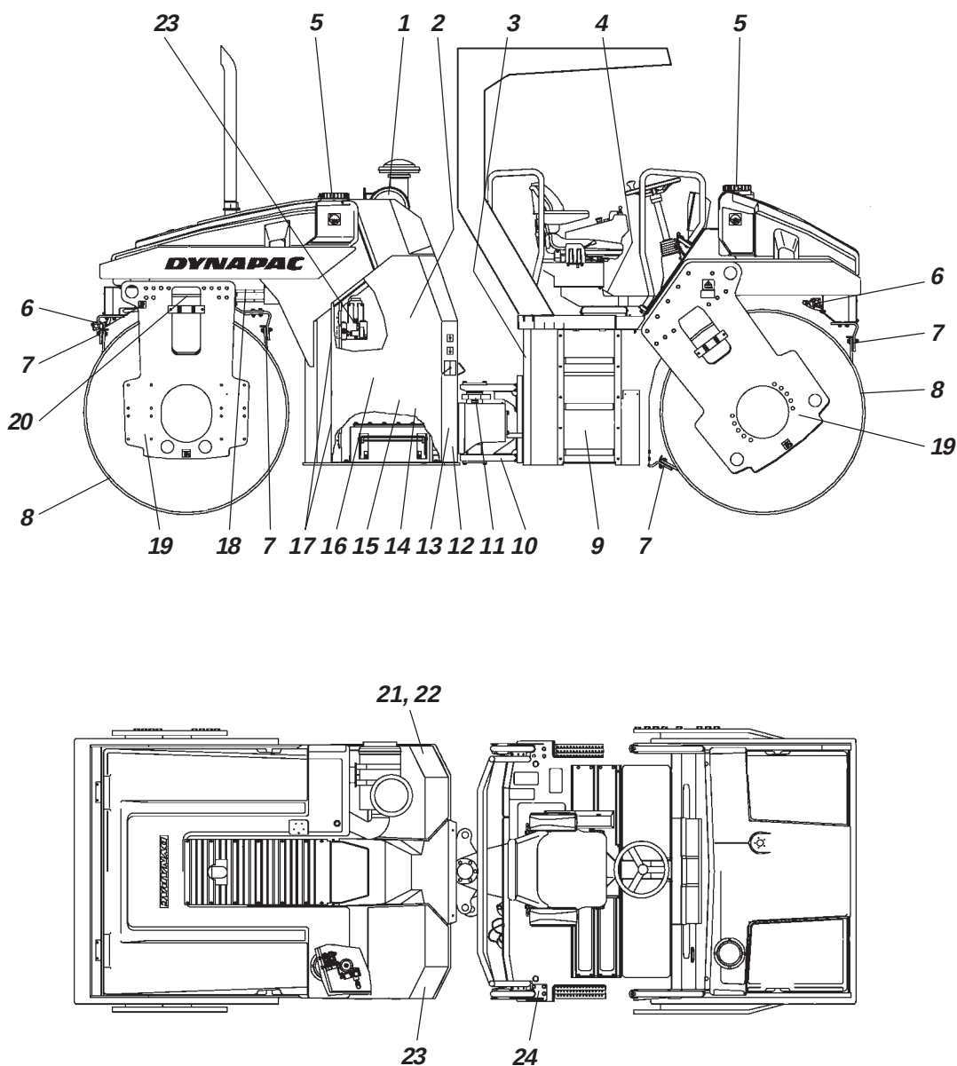
Afb. 1 Service- en onderhoudspunten
