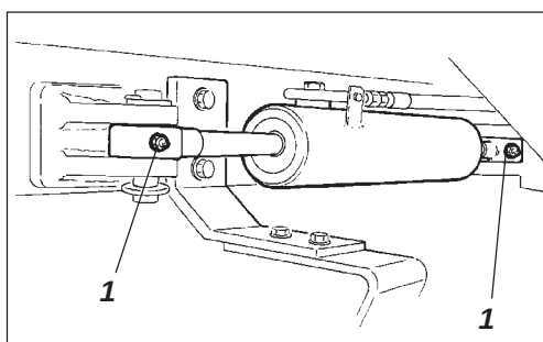
Afb. 16 Draaicylinder 1. Smeernippels
