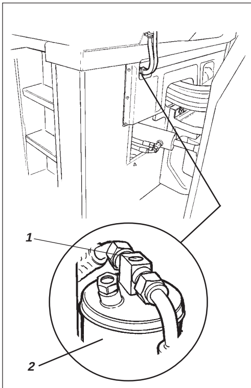
Afb. 21 Droogfilter 1. Kijkglas 2. Filterreservoir
