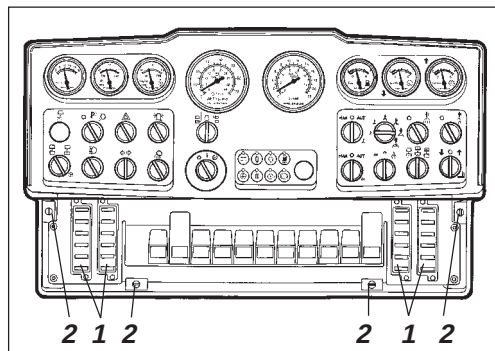
Afb. 54 Instrumentenpaneel
