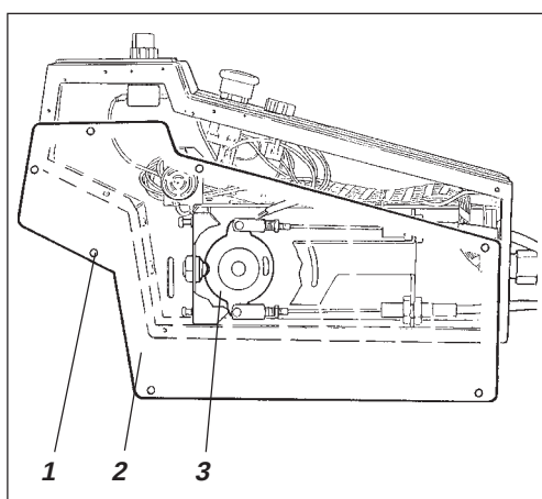
Afb. 47 Vooruit-/achteruithendel
