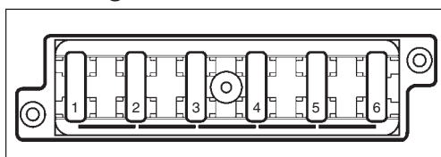
Afb. 60 Zekeringenkast in cabinedak
