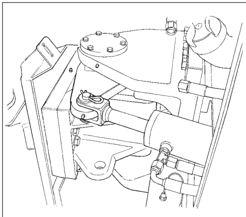
Afb. 48 Stuurverbinding
