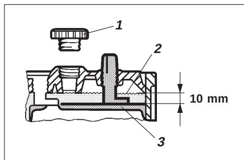
Afb. 25 Vloeistofpeil in accu
