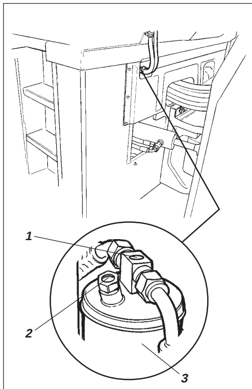
Afb. 52 Droogfilter, onder cabine
