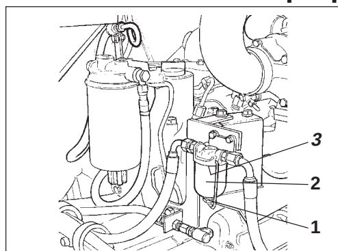
Afb. 36 Dieselmotor
