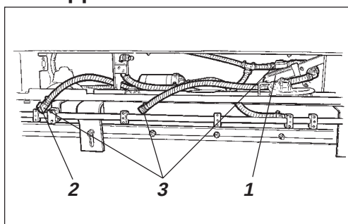
Afb. 45 Pompsysteem
