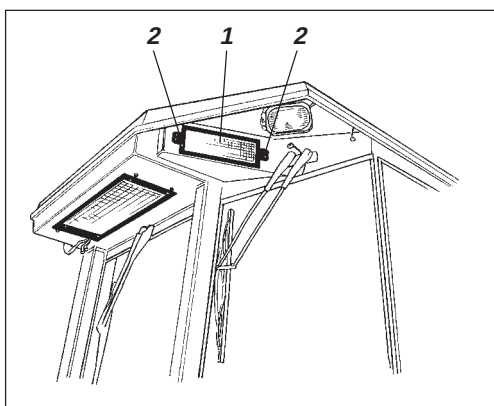
Afb. 40 Cabine 1. Luchtfilter (x2) 2. Schroef (x2)
