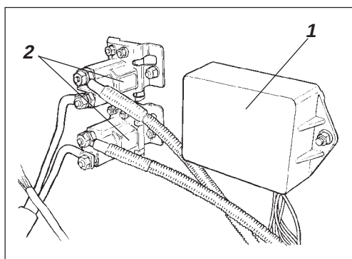
Afb. 57 Motorruimte linkerkant
