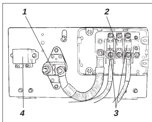
Afb. 56 Hoofdzekeringenpaneel
