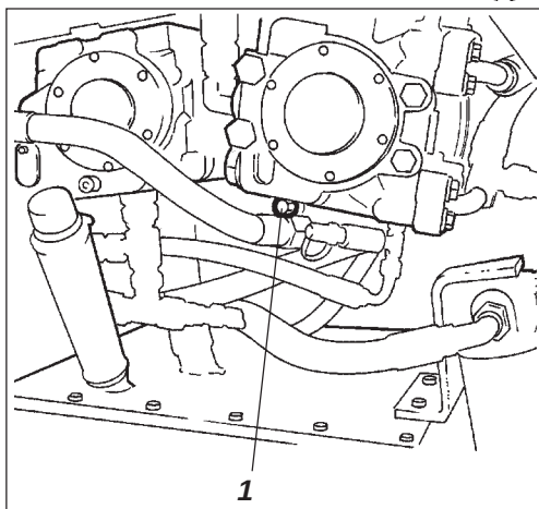
Afb. 39 Pompoeverbrenging 1. Aftapplug
