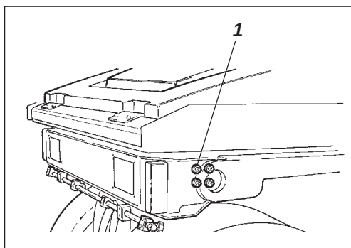
Afb. 30 Achterste wals, rechterkant 1. Smeernippels 4 stuks
