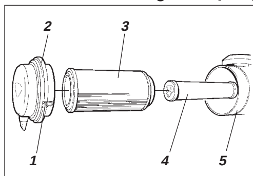
Afb. 17 Luchtfilter
