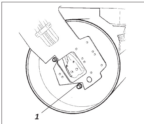
Afb. 41 Wals trillingkant 1. Aftapplug
