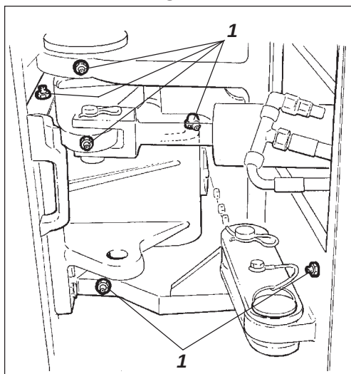
Afb. 14 Rechterzijde van de stuurverbinding 1. Smeernippels
