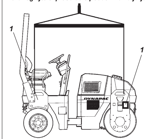
Slika 31 Dviganje valjarja
