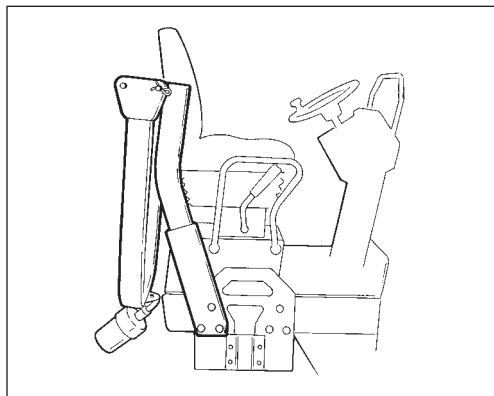
Fig. 39 Struktura ROPS z možnostjo snetja
