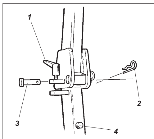
Slika 40 Namestitev zaščitne strukture
