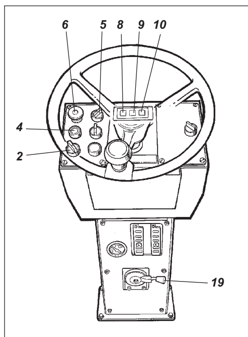
Slik 18 Pult z inštrumenti
