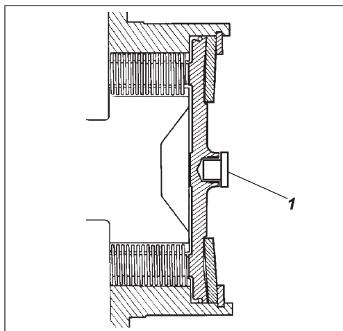
Slika 36 Ohišje zavore
