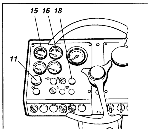
Fig. 15 Vänster instrumentpanel 11. NÖDSTOPP 15. Hydrauloljetemperatur 16. Motortemperatur 18. Varningslampa/luftfilter
