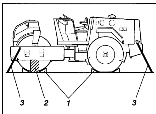
Fig. 32 Transport 1. Bromsblock 2. Uppallning av ramen 3. Spännwire
