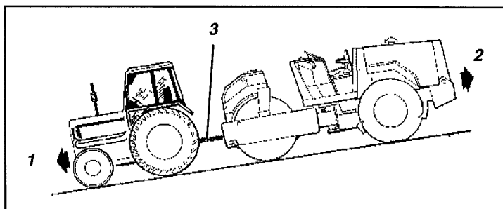
Fig. 30 Motbromsning 1. Färdriktning 2. Motbromsning 3. Bogserstång
