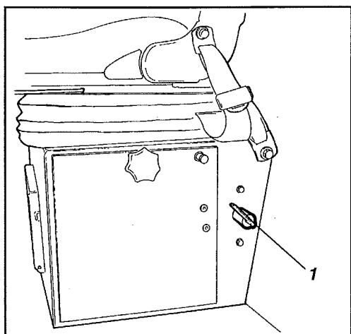
Fig. 23 Batterilåda 1. Batterifrånskiljare
