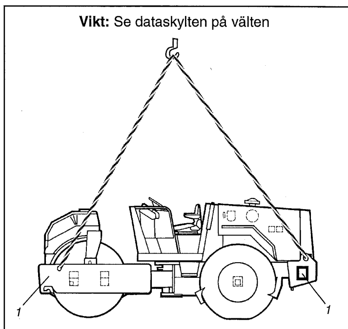
Fig. 26 Lyftning av vält 1. Lyftskylt (främre skylt på höger sida)
