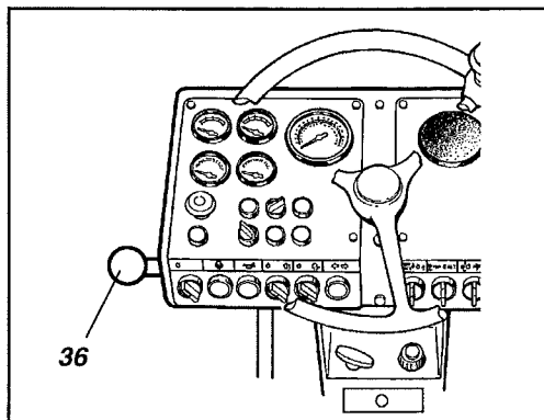
Fig. 16 Instrumentpanel 36. Spak-Avjämnarblad
