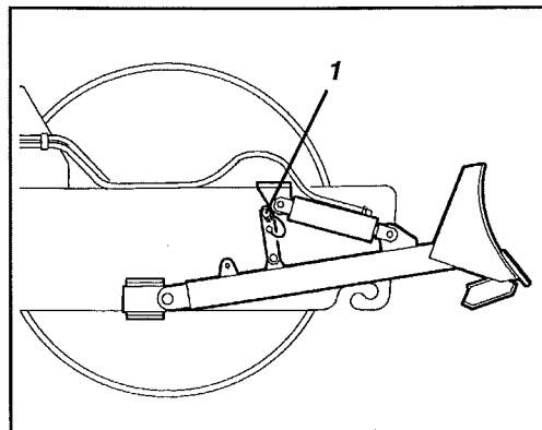
Fig. 11 Avjämnarblad
