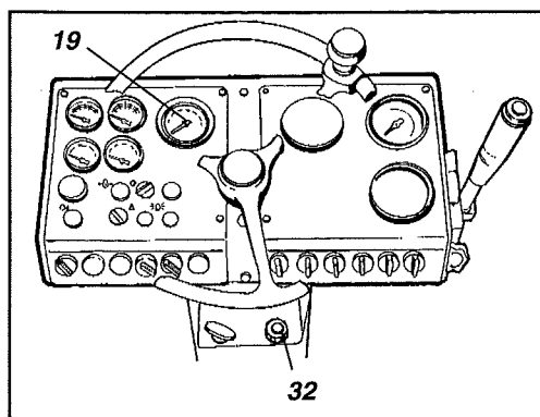
Fig. 13 Instrumentpanel 19. Varv/timräknare 32. Varvtalsreglage
