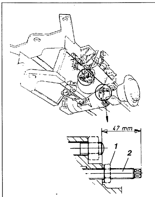
Fig. 29 Bakre axel 1. Låsmutter 2. Skruv
