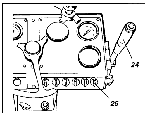
Fig. 14 Höger instrumentpanel 24. Fram/backreglage 26. Hastighetsväljare
