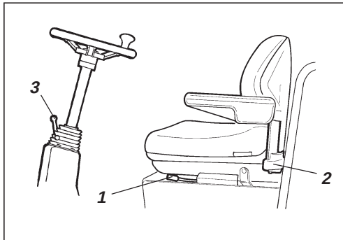
Fig. 11 Assento do operador 1. Alavanca de bloqueio – ajuste longitudinal 2. Manípulo – ajuste do peso 3. Alavanca de bloqueio – inclinação do volante
