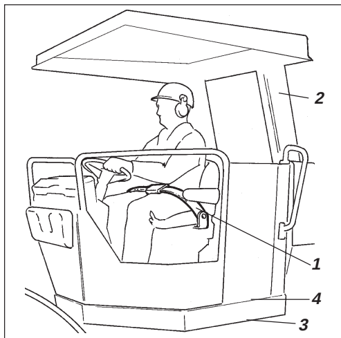
Fig. 16 Lugar do operador 1. Cinto de segurança 2. Arco ROPS 3. Elemento de borracha 4. Proteção contra escorregamento
