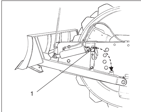
Fig.3 Lâmina niveladora 1. Cavilha de segurança
