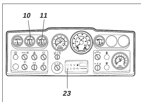
Fig. 23 Painel de instrumentos 10. Temperatura do óleo hidráulico (Acessório) 11. Temperatura do óleo do motor (Acessório) 23. Filtro do ar
