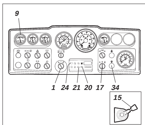
Fig. 20 Painel dos instrumentos 1. Comutador de arranque 9. Voltímetro (Acessório) 15. Regulador de rotação 17. Selector de amplitude 20. Lâmpada dos travões 21. Lâmpada da pressão do óleo 24. Lâmpada de carga da bateria 34. Lâmpada do pré-aquecimento
