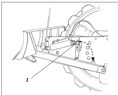
Fig. 18 Lâmina niveladora 1. Cavilha de segurança
