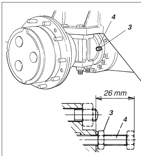
Fig. 37 Eixo traseiro 3. Porca de segurança 4. Parafuso de ajuste
