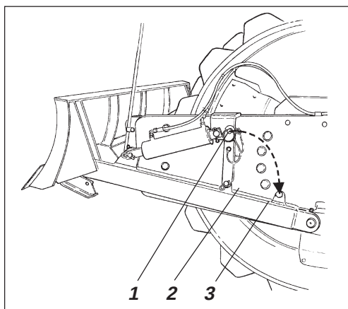
Fig. 27 Lâmina niveladora 1. Cavilha de segurança 2. Tirante de segurança 3. Suporte de estacionamento
