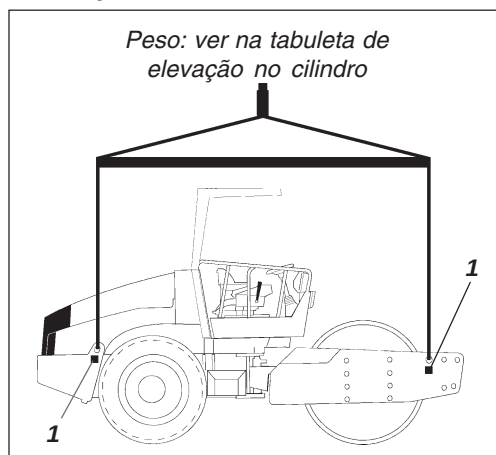
Fig. 34 Cilindro pronto a ser elevado
