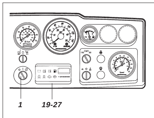
Fig. 30 Painel de instrumentos 1. Comutador de arranque 19-27. Painel de lâmpadas de aviso
