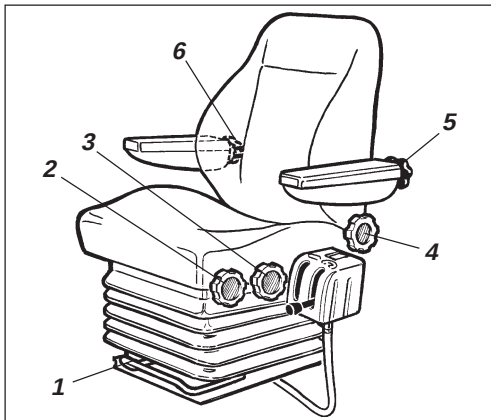
Fig. 13 Assento do operador
