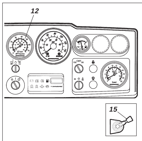
Fig. 21 Painel de instrumentos 12. Conta-rotações (Acessório) 15. Regulador da rotação
