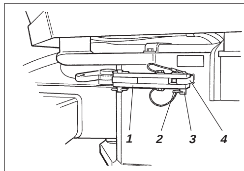
Fig. 35 Articulação da direcção na posição aberta
