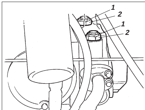
Fig. 36 Bomba de propulsão 1. Válvula de reboque 2. Porca de segurança
