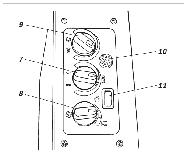
Fig. 9c Cabina, lado direito (com acessório AC)
