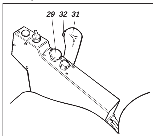
Fig. 29 Painel de comandos 29. Comando do travão de reserva/ estacionamento 31. Comando Avanço/Recuo 32. Interruptor vibração Ligado/ Desligado
