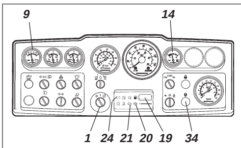
Fig. 14 Painel de instrumentos
