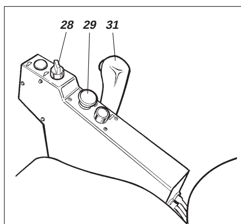
Fig. 22 Painel de comandos 28. Selector de velocidade, eixo traseiro 29. Botão do travão de Reserva/Estacionamento 31. Comando de Avanço/Recuo
