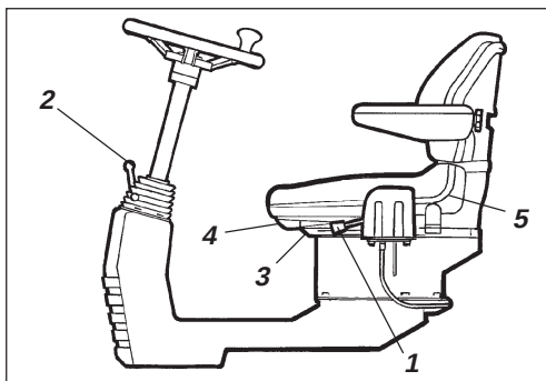
Fig. 12 Lugar do operador 1. Alavanca de bloqueio – rotação (Acessório) 2. Alavanca de bloqueio – inclinação do volante 3. Alavanca de bloqueio – ajuste longitudinal 4. Manípulo – inclinação do encosto 5. Manípulo – ajuste do peso
