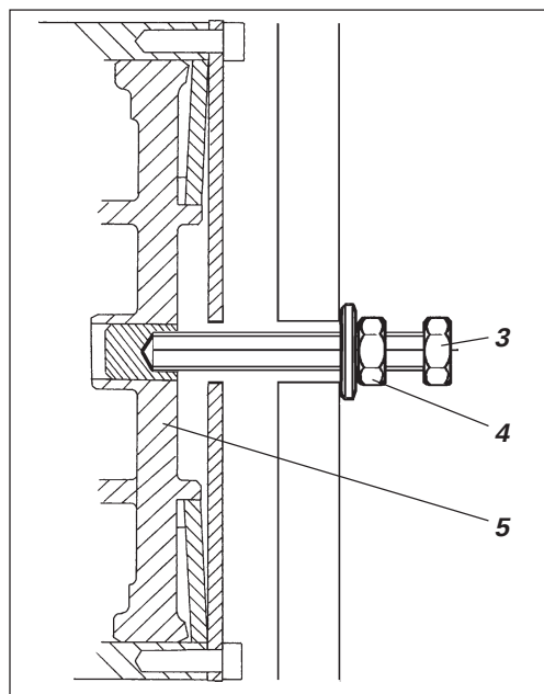
Fig. 39 Corte transversal da caixa do travão
