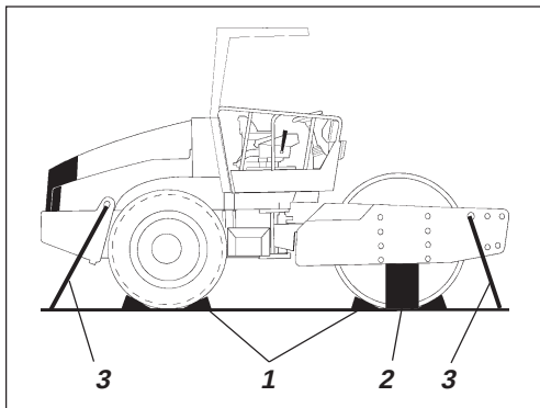
Fig. 41 Transporte
