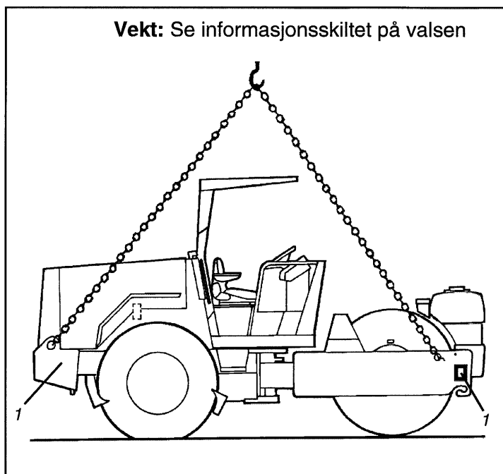
Fig. 26 Løfting av vals 1. Løfteskilt (bakre skilt på venstre side)
