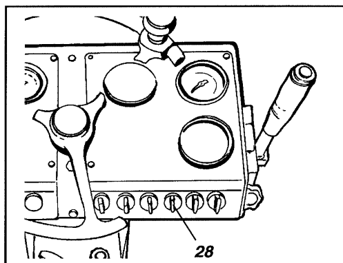
Fig. 17 Høyre instrumentpanel 28. Utslagsvelger
