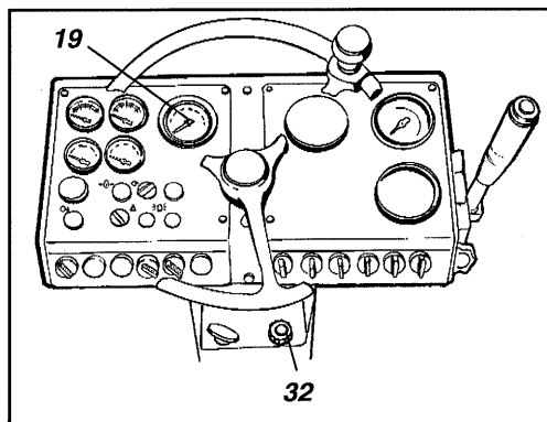
Fig. 13 Instrumentpanel 19. Tur-/tidsteller 32. Bryter for turtall
