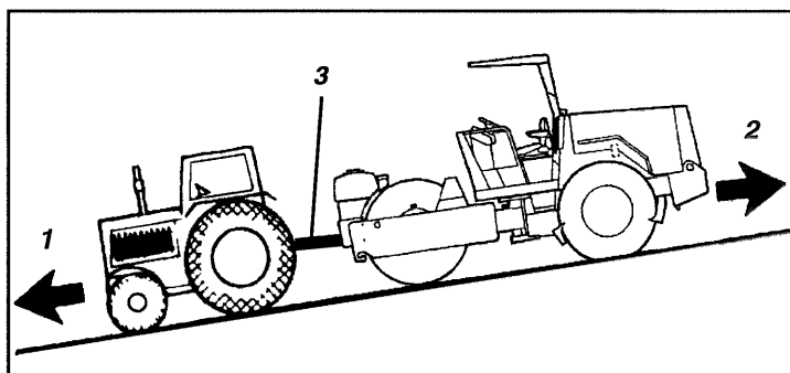
Fig. 30 Motbremsing
