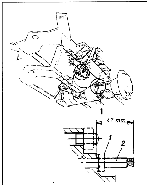
Fig. 29 Bakaksel
