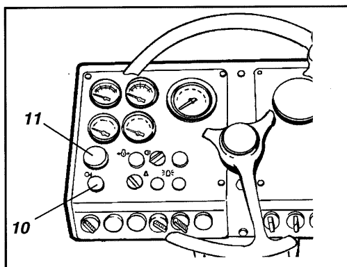
Fig. 24 Venstre instrumentpanel 10. Varsellampe for brems 11. NØDSTOPPBryter
