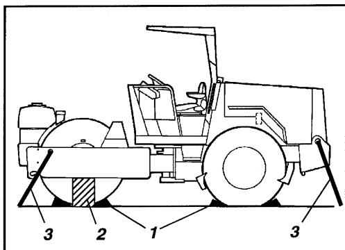
Fig. 32 Transport 1. Blokk 2. Blokkering 3. Spennwire
