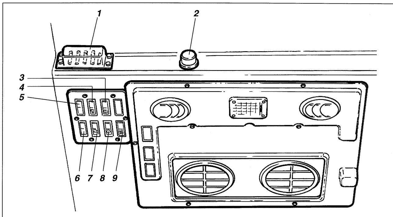
Fig. 5 Taket i førerhuset
