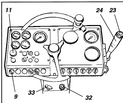
Fig. 21 Instrumentpanel 9. Startstrømbryter (Stopp - Cummins) 11. NØDSTOPPBryter 23. Vibrasjon På/Av 24. Forover-/bakoverspake 32. Bryter for turtall 33. Stoppbryter (Deutz)
