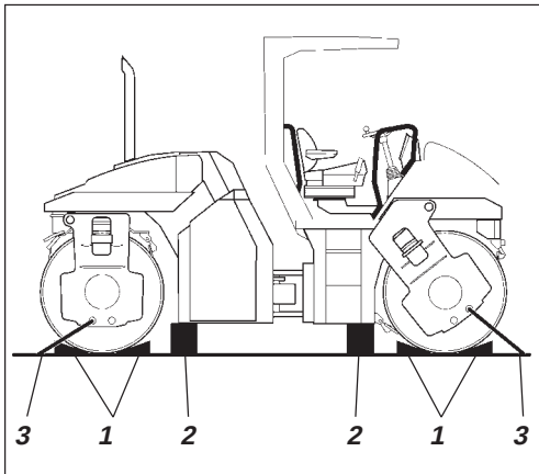
Fig. 40 Transport av vält
