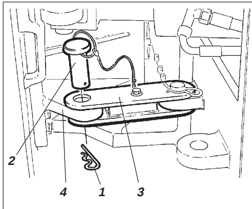
Fig. 32 Styrled i låst läge
