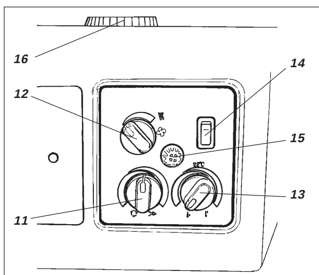
Fig. 9d Hytt, med AC (tillbehör)
