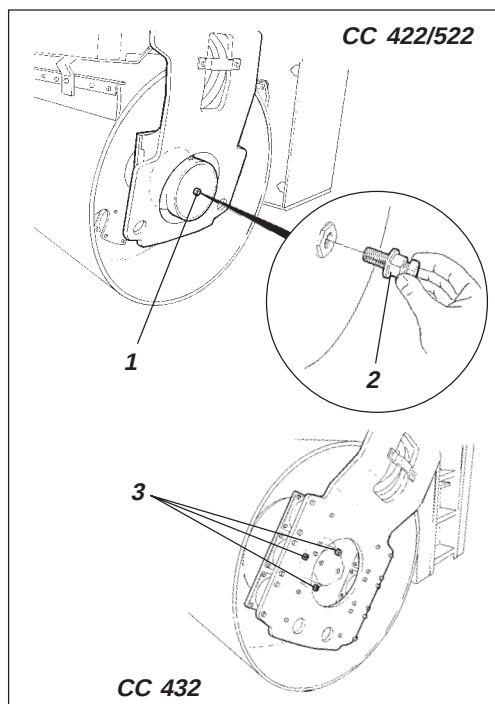
Fig. 36 Valsdrivningsmotor 1. Centrumplugg 2. M16x100 samt bricka och mutter 3. Pluggar (3st) för bromsfriläggning
