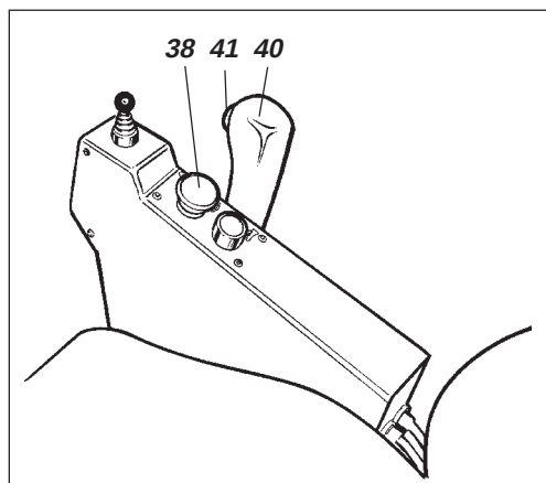
Fig. 28 Reglagepanel 38. Reserv/parkeringsbromsknapp 40. Fram/Backreglage 41. Strömbrytare vibration Till/Från
