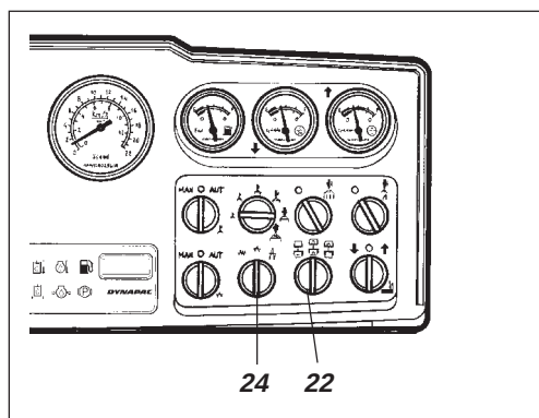
Fig. 24 Instrumentpanel 22. Strömbrytare valsar 24. Strömbrytare Hög/Låg
