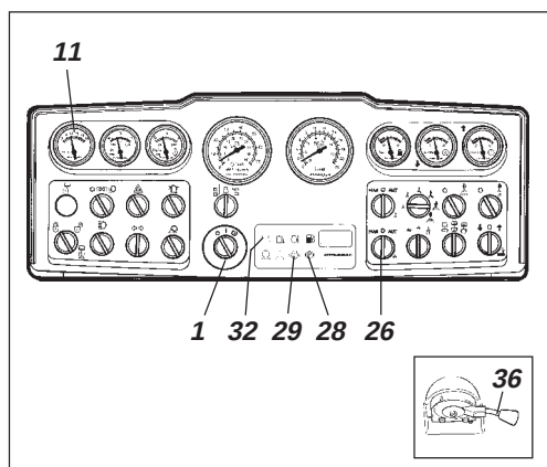
Fig. 18 Instrumentpanel 1. Startströmbrytare 11. Voltmätare (tillbehör) 26. Vibrationsströmbrytare 28. Bromsvarningslampa 29. Oljetryckslampa 32. Laddningslampa 36. Varvtalsreglage
