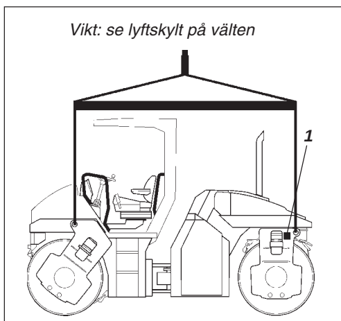
Fig. 33 Vält förberedd för lyft
