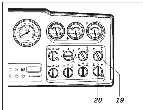
Fig. 25 Omkopplare
