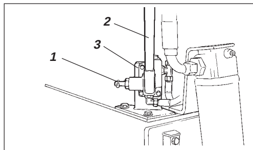
Fig. 37 Bromsfriläggingspump
