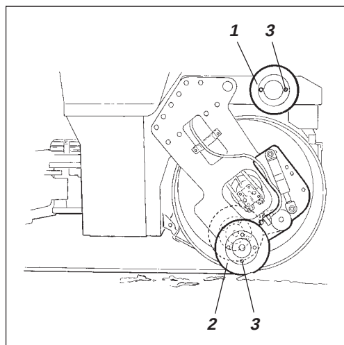
Fig. 26 Byte av verktyg
