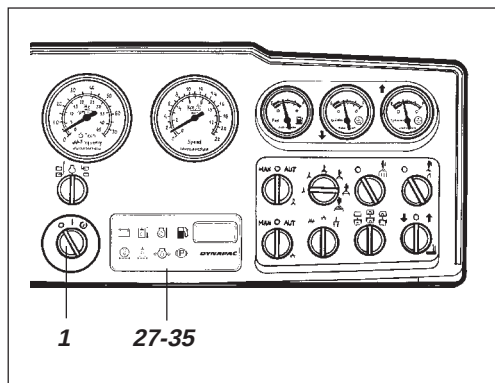
Fig. 29 Instrumentpanel 1. Startströmbrytare 27-35. Panel för varningslampor
