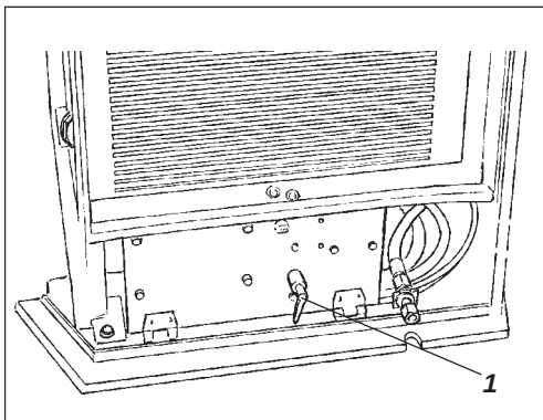
Fig. 31 Motorutrymme 1. Batterifrånskiljare
