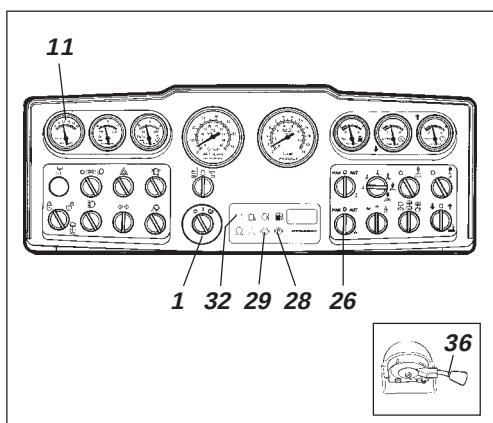
Fig. 17 Instrumentpanel 1. Startafbryder 11. Voltmeter (ekstraudstyr) 26. Vibrationsafbryder 28. Bremselampe 29. Olietryklampe 32. Ladelampe 36. Omdrejningstalsregulering
