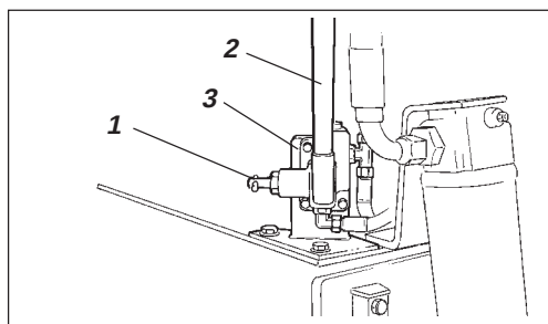
Fig. 34 Bremsefrilægningspumpe
