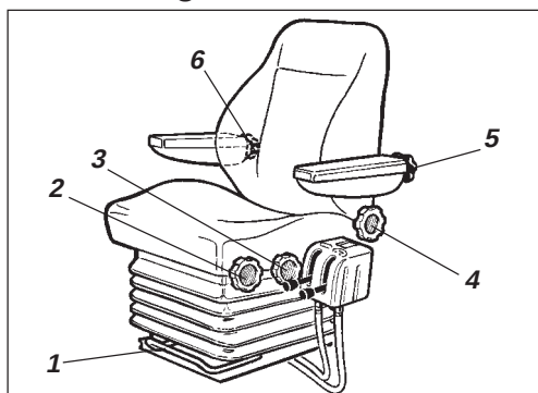
Fig. 11 Førersæde 1. Håndtag – længdeindstilling 2. Drejehåndtag – højdeindstilling 3. Drejehåndtag – sædehældning 4. Drejehåndtag – ryglænhældning 5. Drejehåndtag – armlænhældning 6. Drejehåndtag – indstilling af lændestøtte
