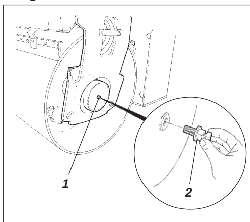
Fig. 33 Valsedriftsmotor 1. Centerprop 2. M16x100 samt skive og møtrik
