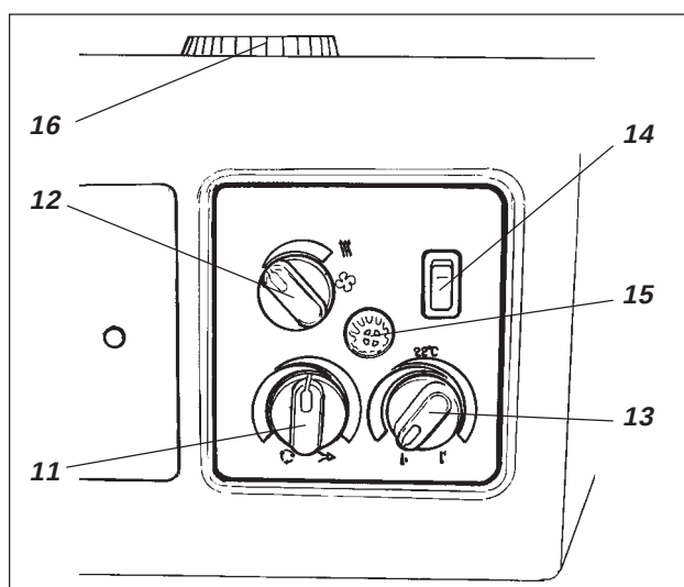
Fig. 8d Førerhus med AC (ekstratilbehør)
