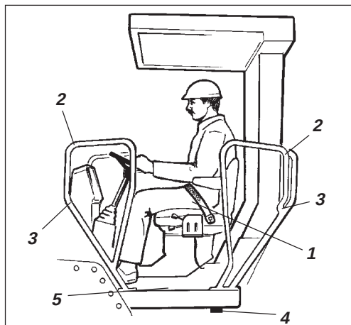
Fig. 15 Førerplads
