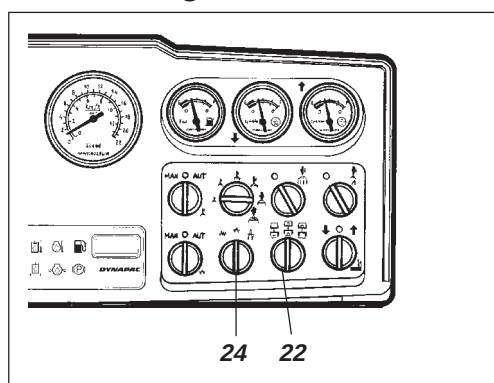
Fig. 23 Instrumentpanel 22. Afbryder, valser 24. Afbryder, Høj/Lav
