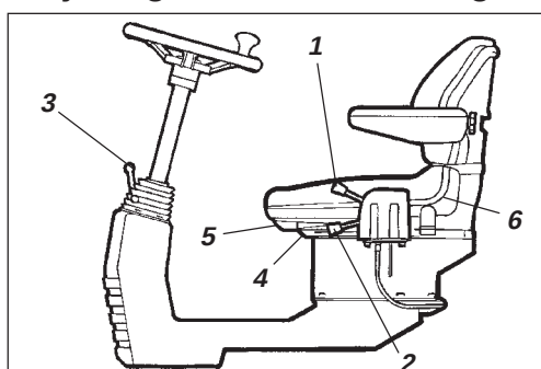
Fig. 10 Førerplads 1. Låsehåndtag – tværgående bevægelse 2. Låsehåndtag – rundsving 3. Låsehåndtag – rathældning 4. Låsehåndtag – længdeindstilling 5. Håndtag – ryglænhældning 6. Håndtag – vægtindstilling
