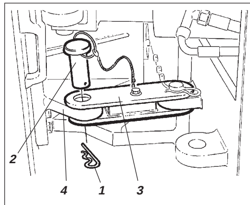
Fig. 29 Styreled i låst stilling
