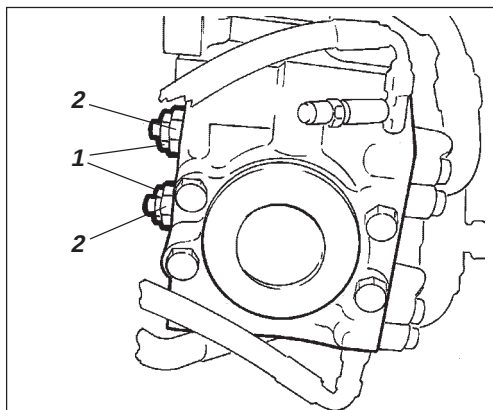
Fig. 32 Fremdrivningspumpe 1. Bugserventil 2. Flerfunktionsventil
