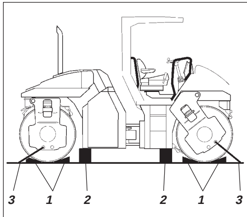
Fig. 37 Transport af tromle
