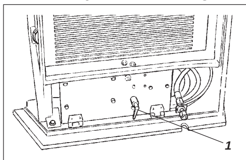
Fig. 9 Motorrum 1. Batteriafbryder
