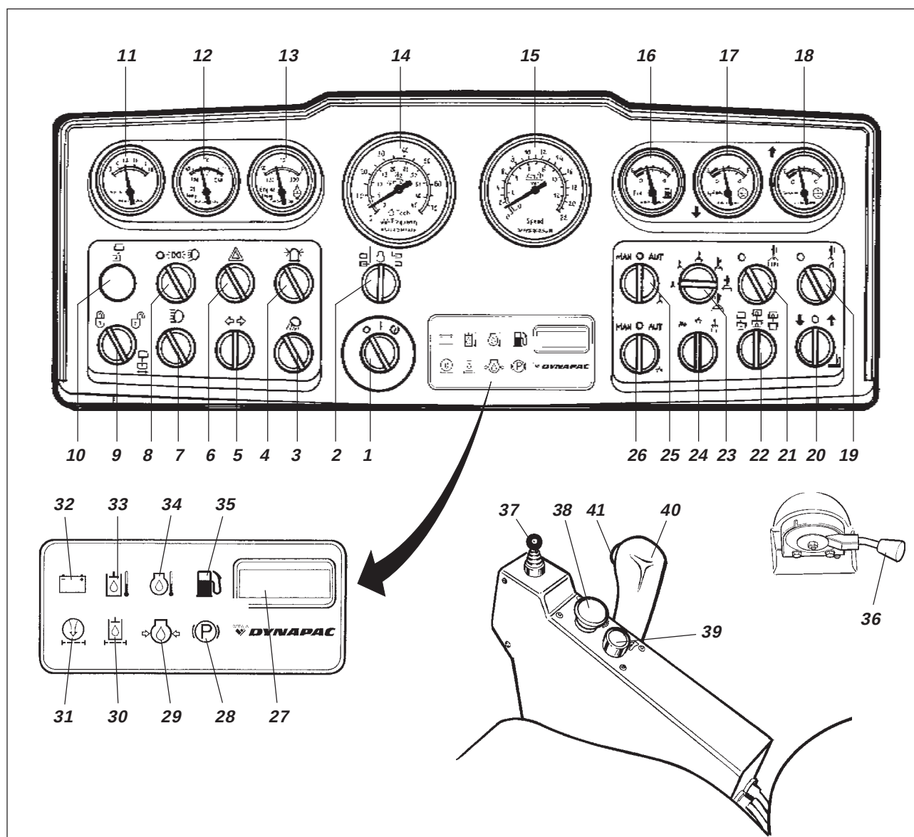
Fig. 7 Instrumenter og betjeningspanel
