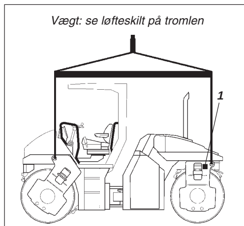
Fig. 30 Tromle forberedt til løftning
