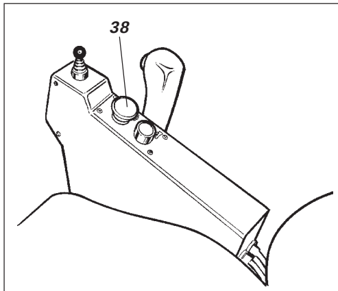
Fig. 24 Reguleringspanel 38. Reserve-/Parkeringsbremseknapp
