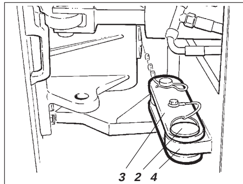
Fig. 31 Styreled i åben stilling
