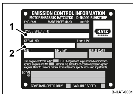
Obr. 2: Typový štítok motora (príklad)
