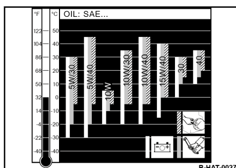
Bild 72: Ölviskositätsdiagramm
