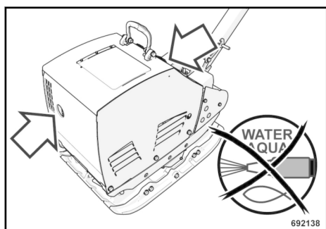
Bild 113: Maschine reinigen (Beispiel)
