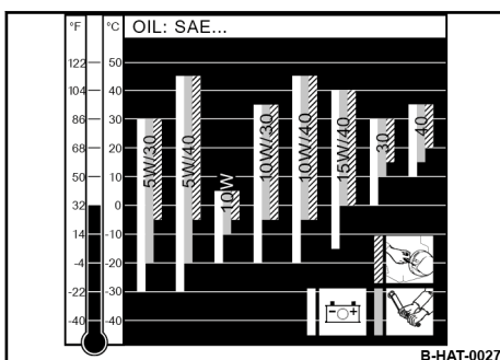
Bild 64: Ölviskositätsdiagramm
