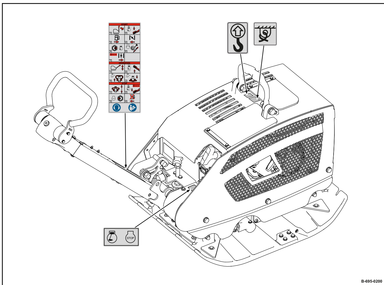
fig. 8: Capot à protection totale (option)
