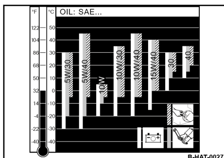
Fig. 73: Diagramma viscosità dell'olio
