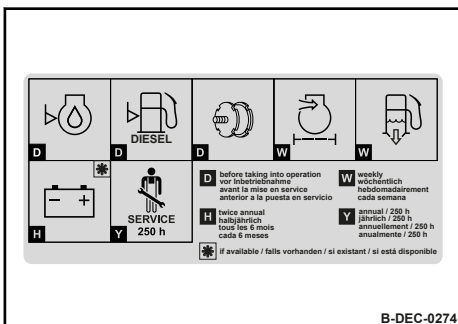
Wartungsschild
