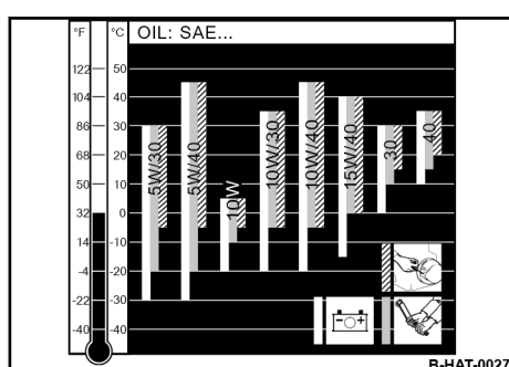
Fig. 63: Diagrama de viscosidad de aceites
